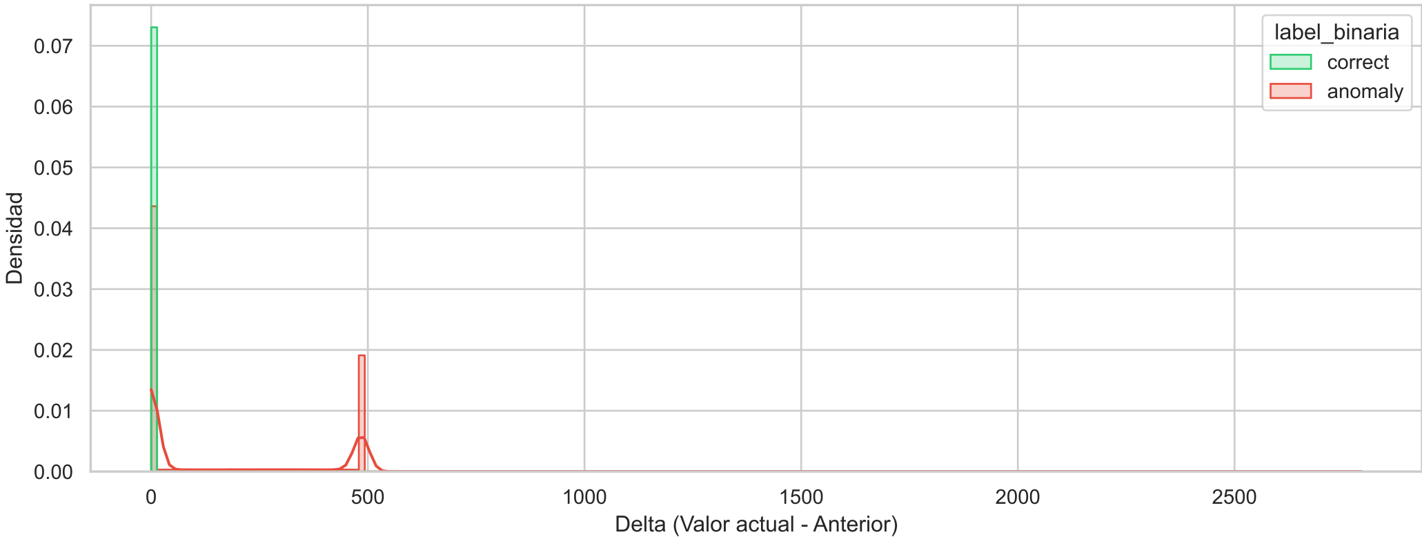
Histograma de Densidad Binario (net_contrack_listener_conn_accepted_total_diff)
