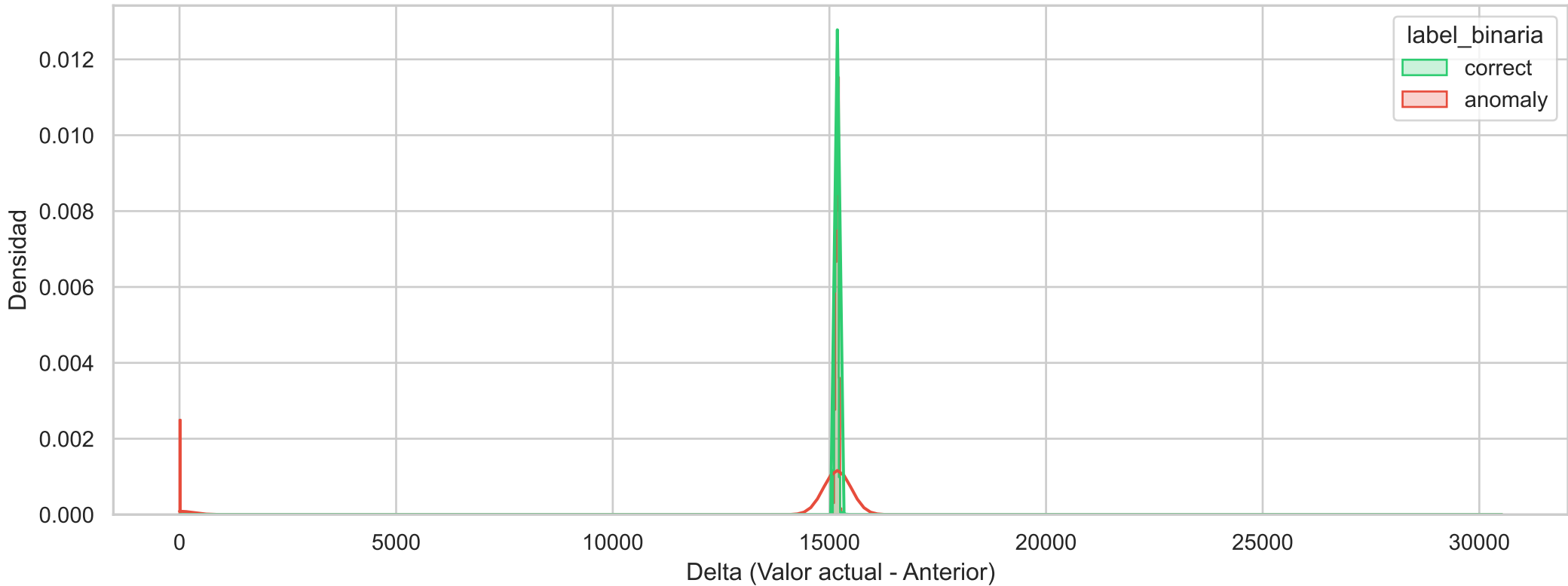
Histograma de Densidad Binario (node_netstat_IpExt_OutOctets_diff)
