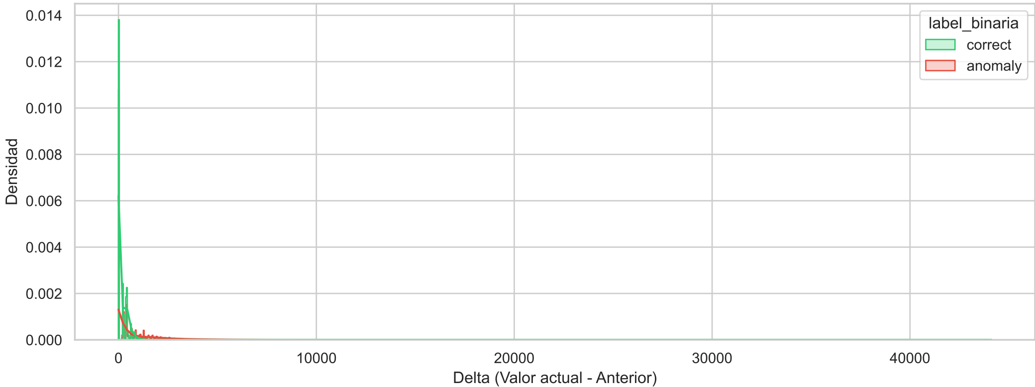
Histograma de Densidad Binario (go_memstats_buck_hash_sys_bytes_diff)
