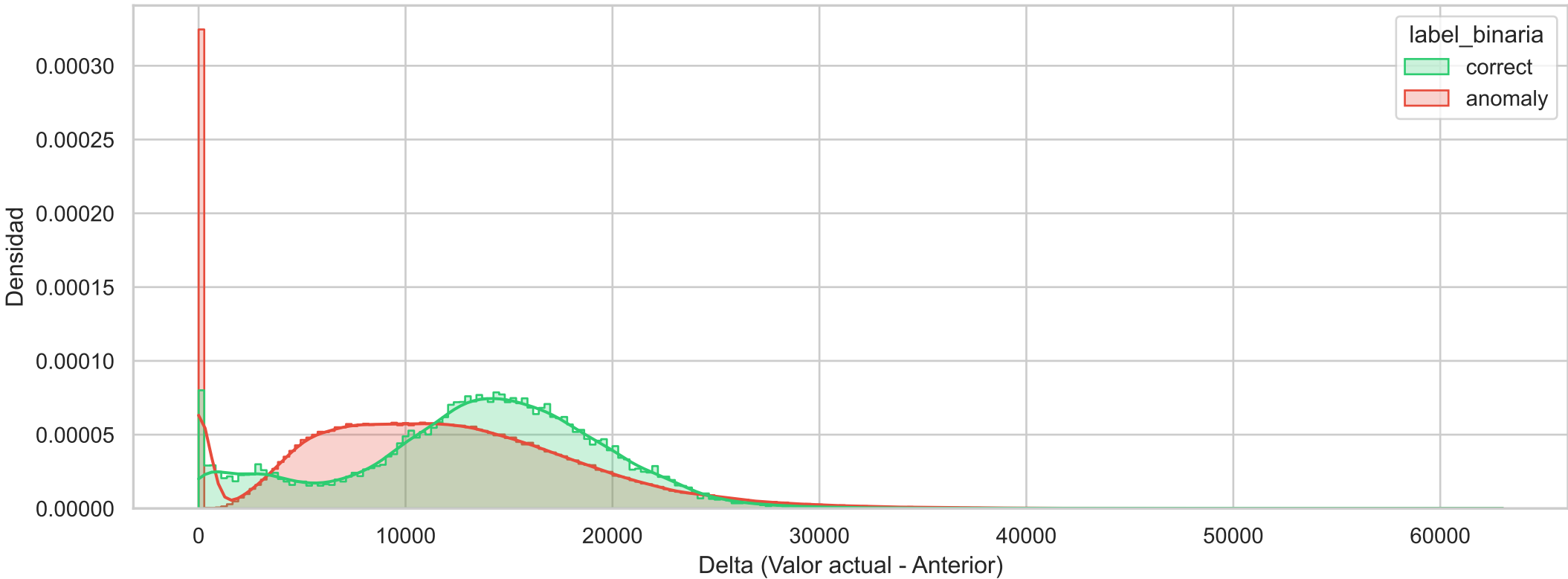
Histograma de Densidad Binario (node_schedstat_timeslices_total_diff)
