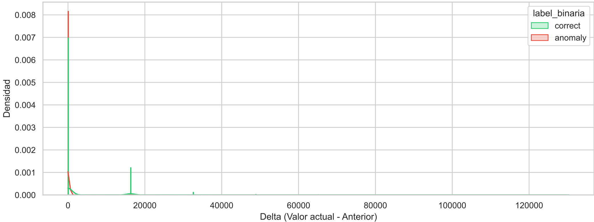
Histograma de Densidad Binario (go_memstats_mspan_sys_bytes_diff)
