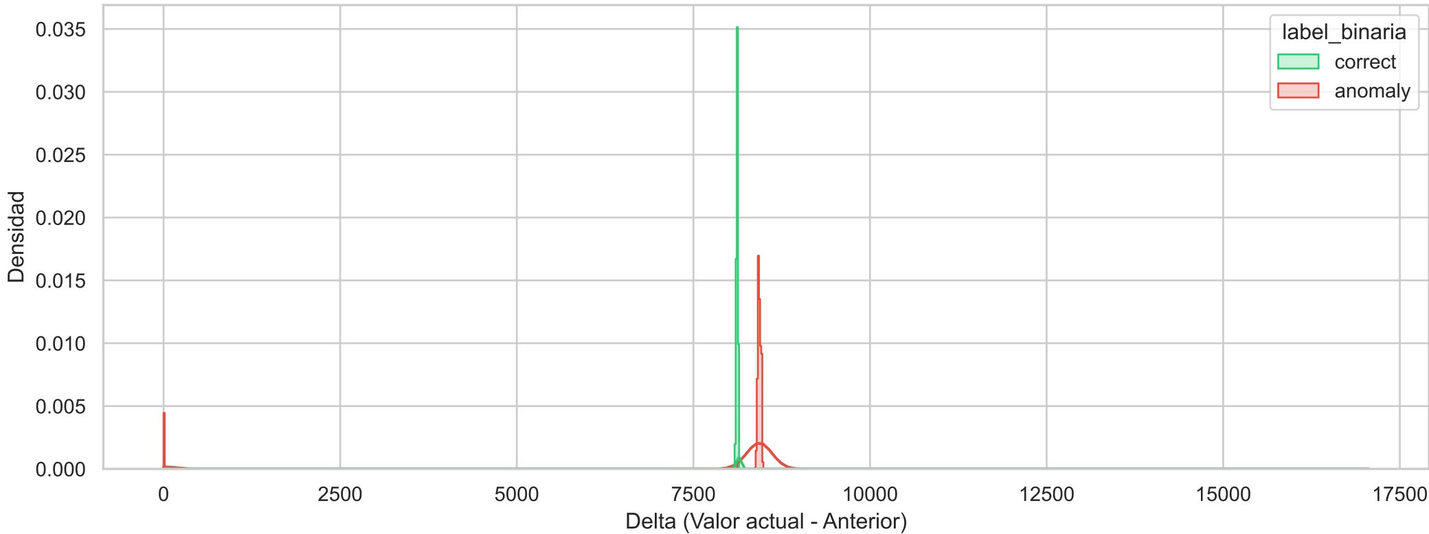
Histograma de Densidad Binario (prometheus_http_response_size_bytes_sum_diff)
