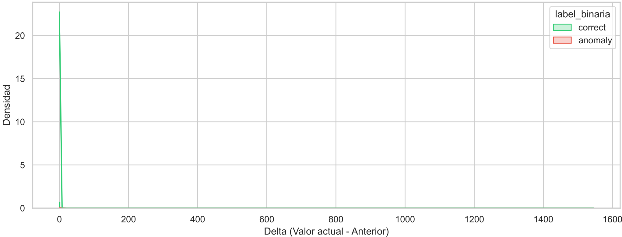
Histograma de Densidad Binario (prometheus_tsdb_head_chunks_diff)
