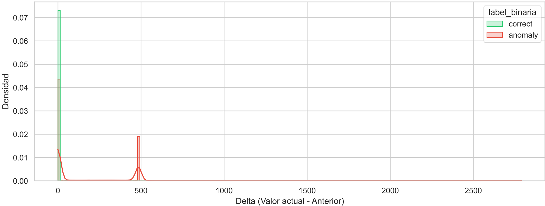
Histograma de Densidad Binario (net_contrack_listener_conn_closed_total_diff)
