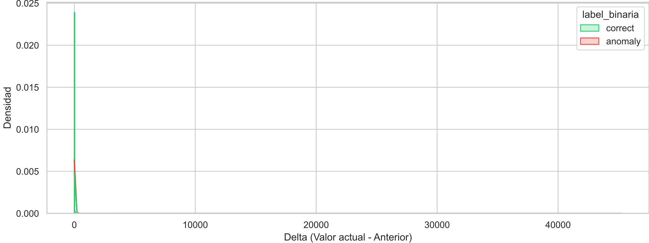
Histograma de Densidad Binario (node_vmstat_pgmajfault_diff)
