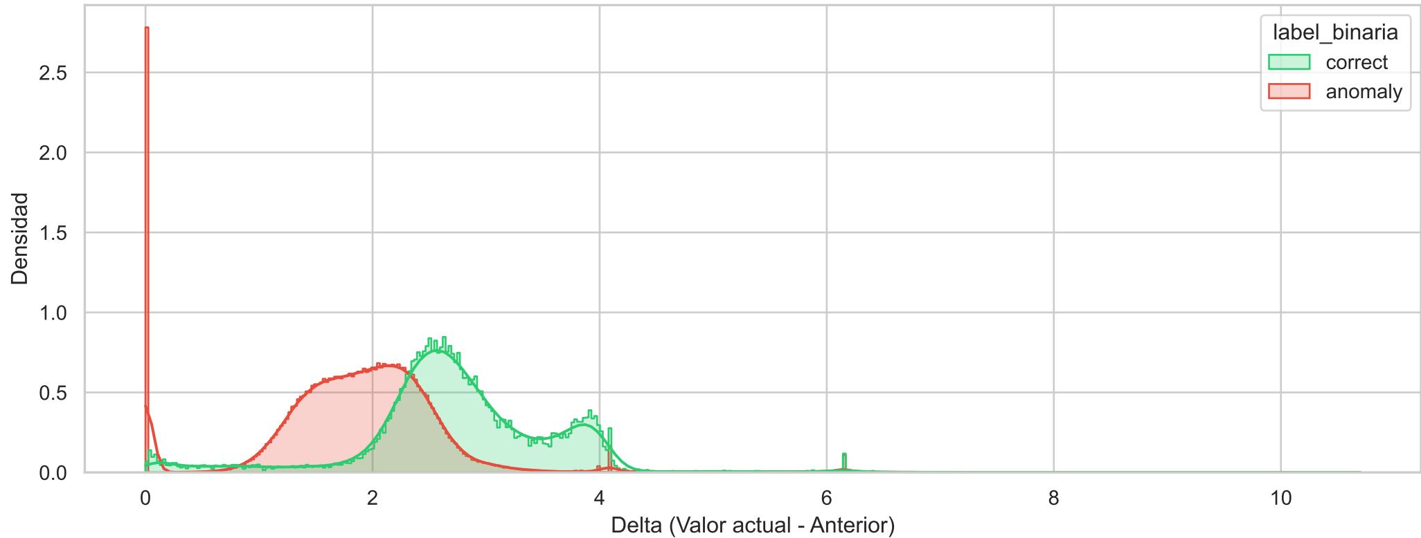
Histograma de Densidad Binario (node_schedstat_running_seconds_total_diff)
