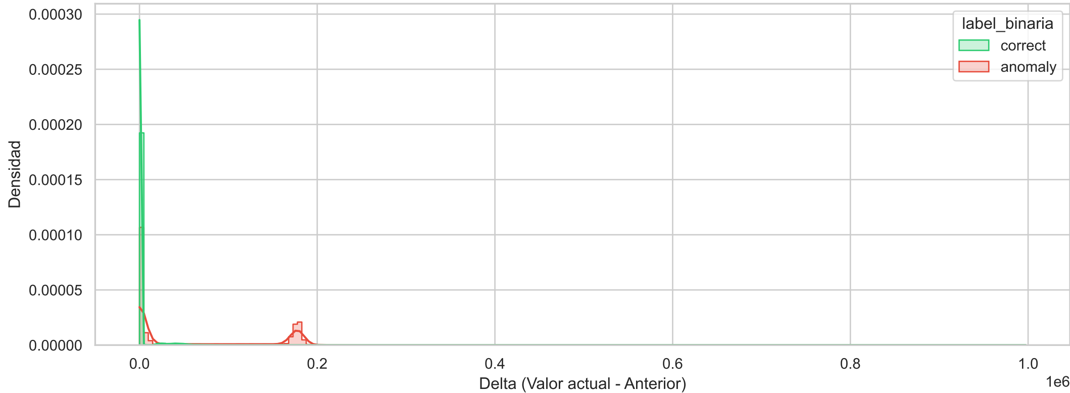
Histograma de Densidad Binario (go_memstats_frees_total_diff)
