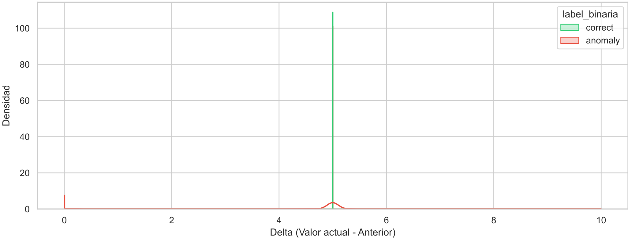
Histograma de Densidad Binario (node_netstat_Tcp_InSegs_diff)
