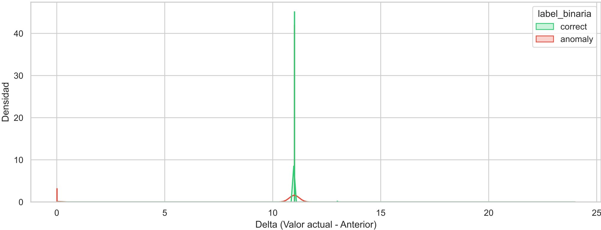
Histograma de Densidad Binario (node_netstat_Tcp_OutSegs_diff)
