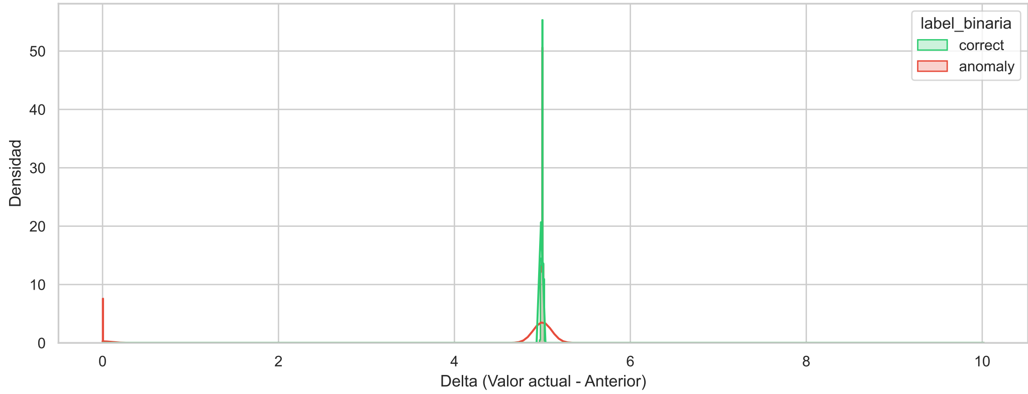
Histograma de Densidad Binario (node_time_seconds_diff)
