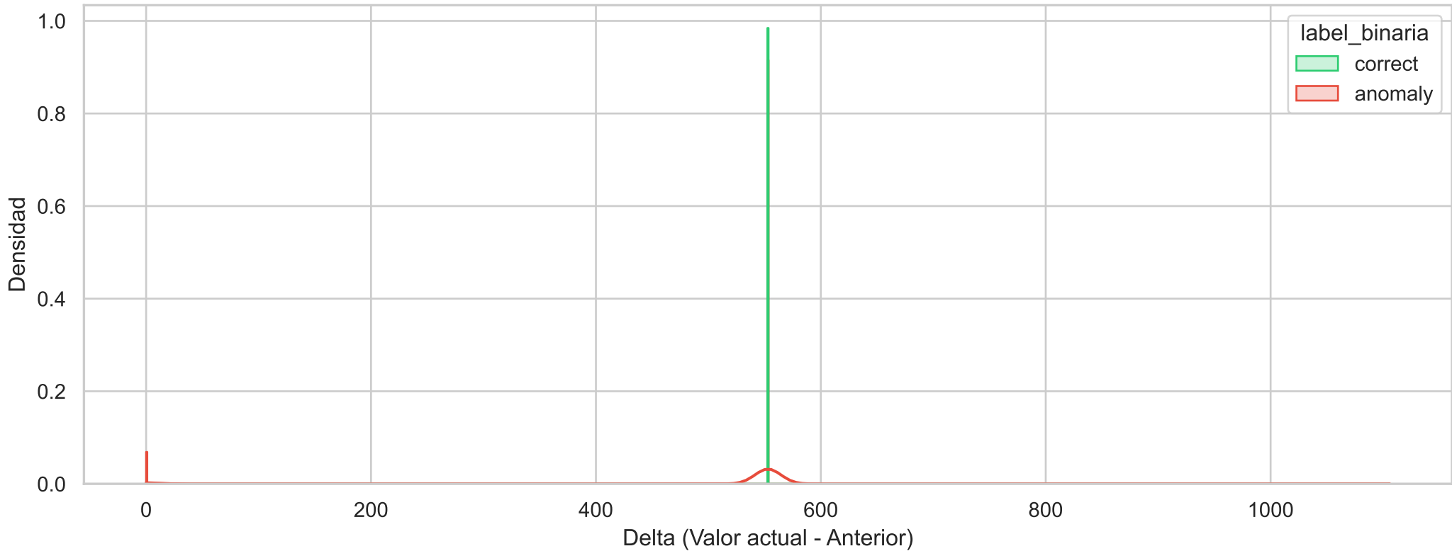
Histograma de Densidad Binario (node_netstat_IpExt_InOctets_diff)
