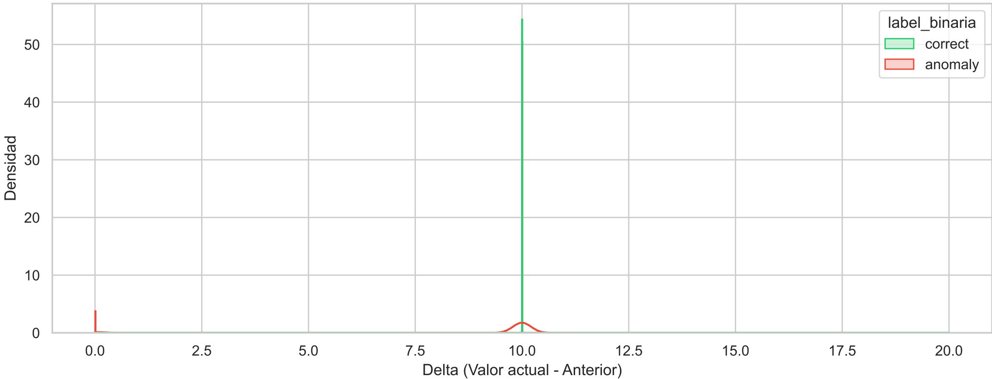
Histograma de Densidad Binario (prometheus_target_interval_length_seconds_sum_diff)
