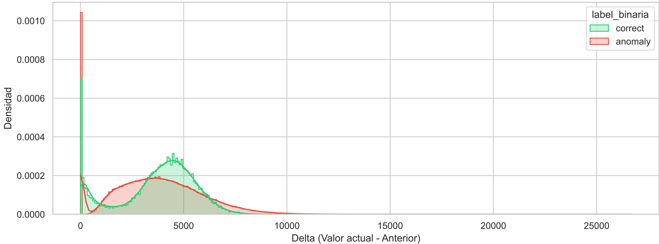
Histograma de Densidad Binario (node_softnet_processed_total_diff)
