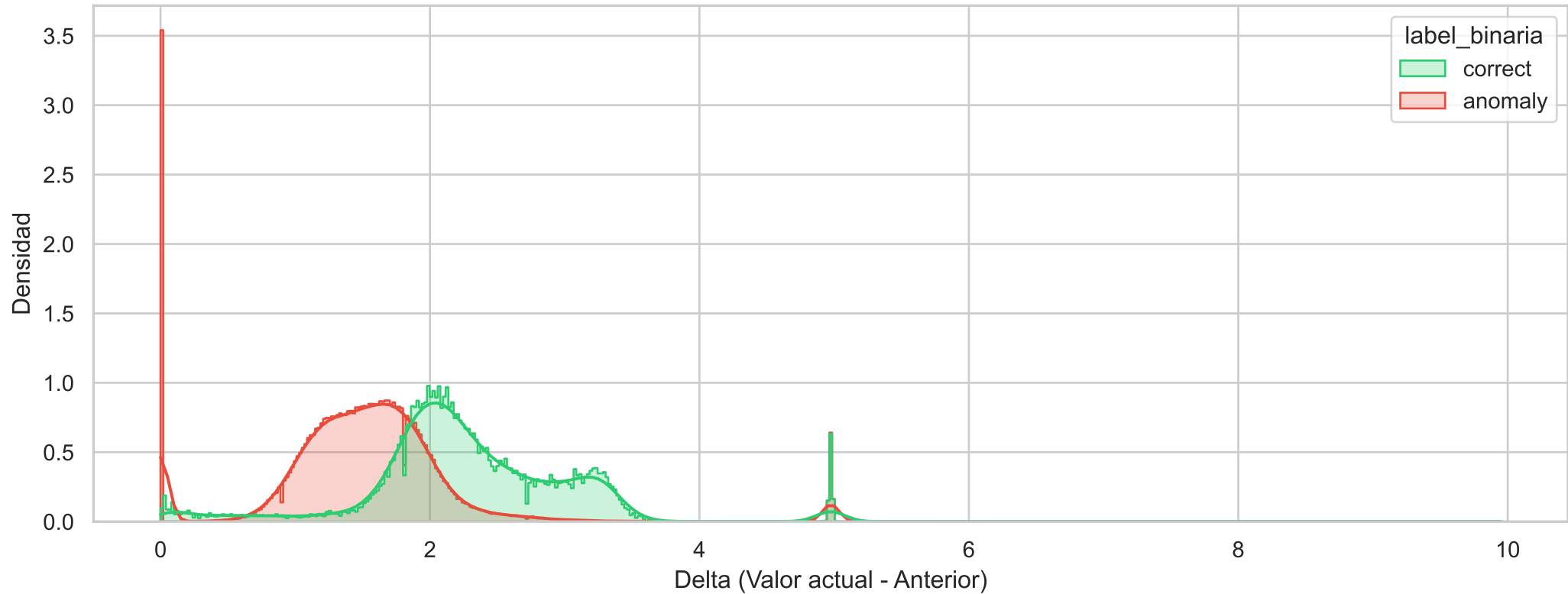
Histograma de Densidad Binario (node_cpu_seconds_total_diff)
