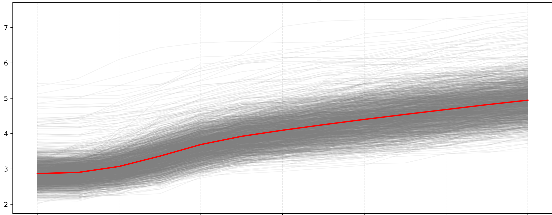
Series Centradas: node_load5
