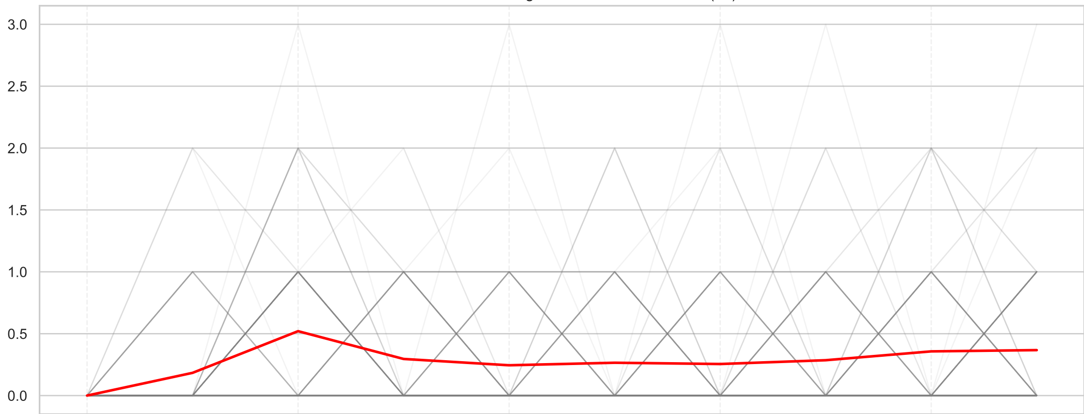
Series Centradas: light-oauth2-oauth2-token-1(35)
