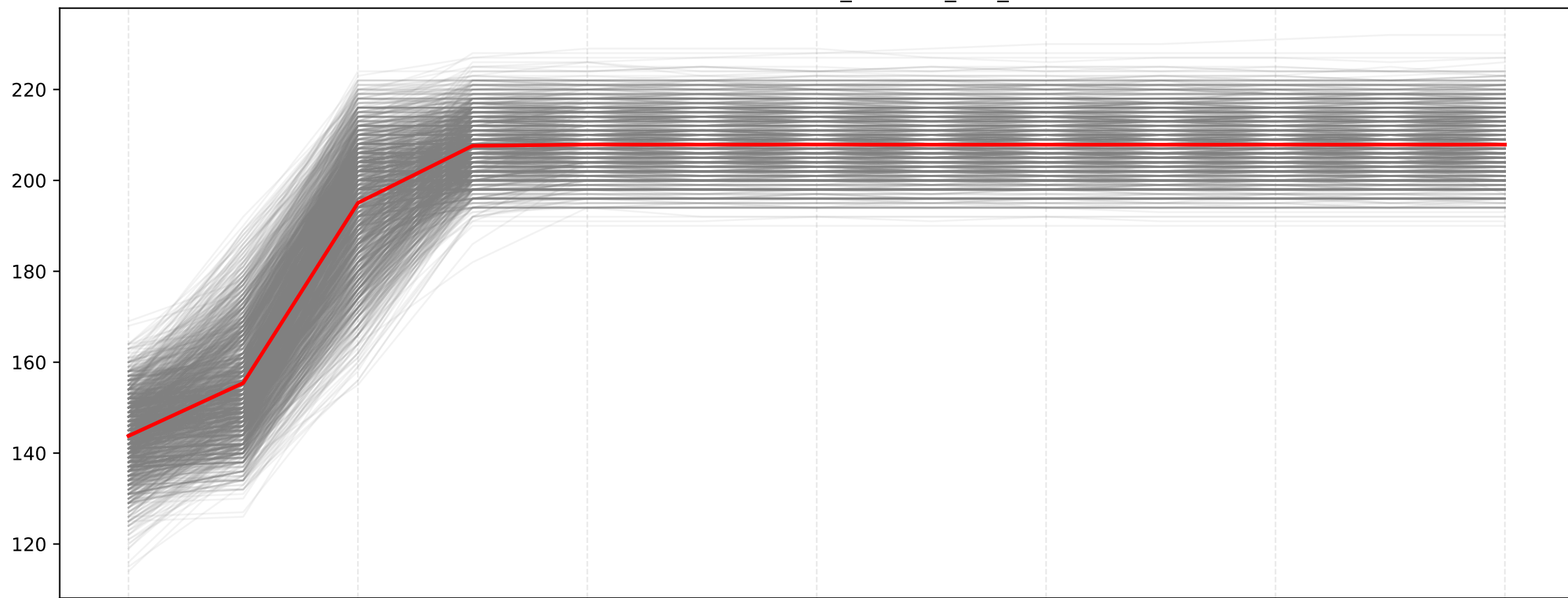
Series Centradas: node_sockstat_TCP_alloc
