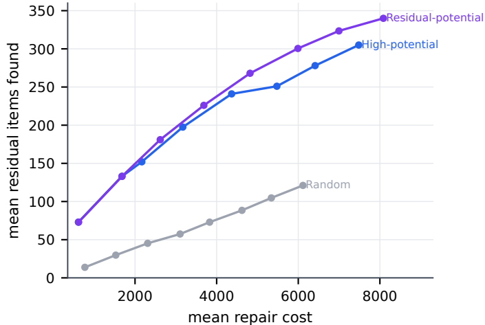
(a) Budget frontier: gain vs cost
