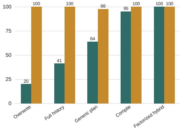
GLM-5.1
