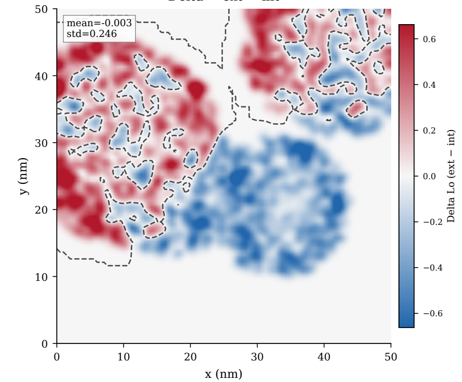
F Asimetría Lo externa vs. interna Delta = ext - int
