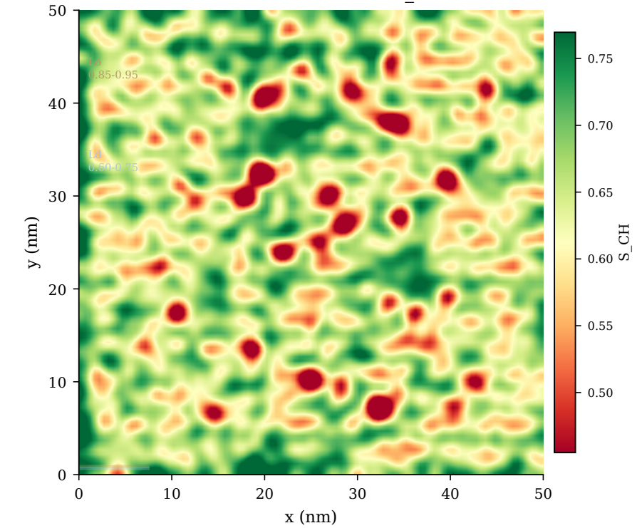
C Parametro de orden S_{CH}
