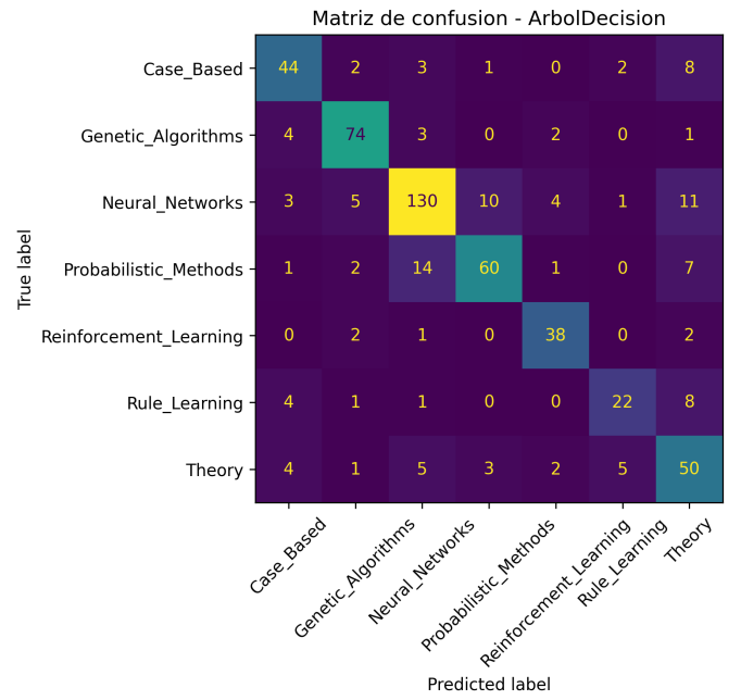
Fig. 5. Matriz de confusión del mejor modelo base (Arbol de Decision, T2.1).
