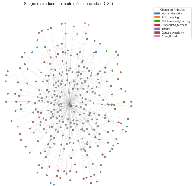
Fig. 4. Subgrafo ego del nodo con mayor conectividad. Ilustra estructura local densa.
