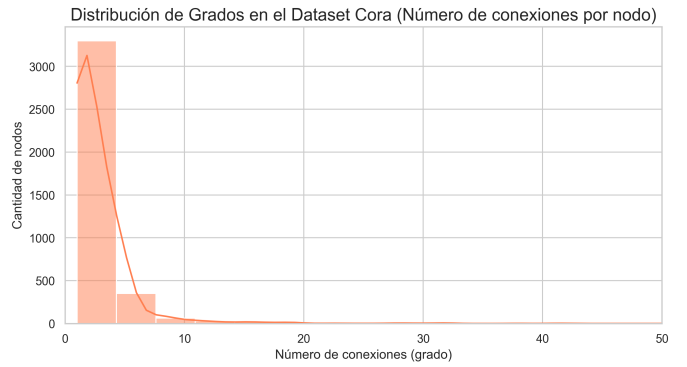
Fig. 3. Distribucion de grados del grafo de citacion Cora.
