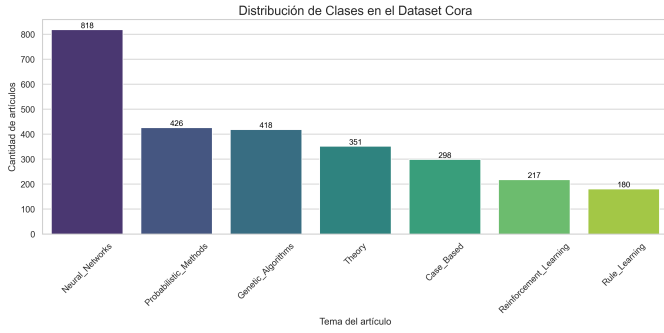
Fig. 1. Distribucion de clases del dataset Cora.
