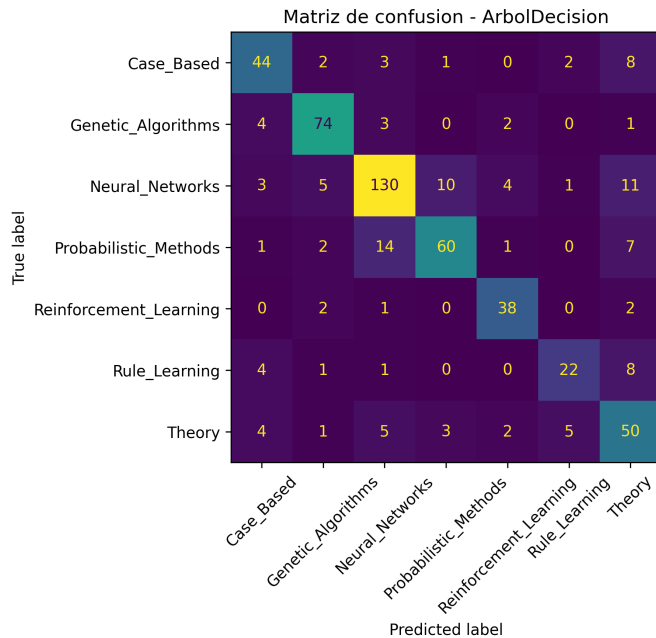
Fig. 9. Matriz de confusión del mejor modelo base (Árbol de Decisión, T2.1).
