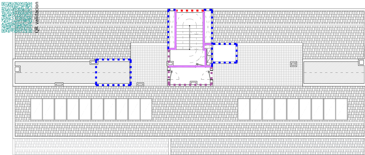
PLANTA BAJO-CUBIERTA
