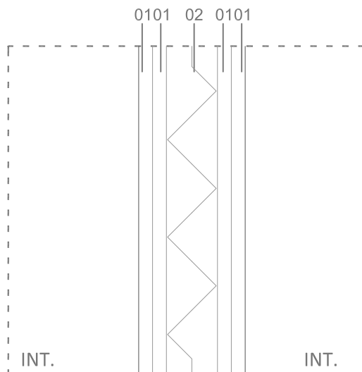
P02: PARTICIÓN INTERIOR
