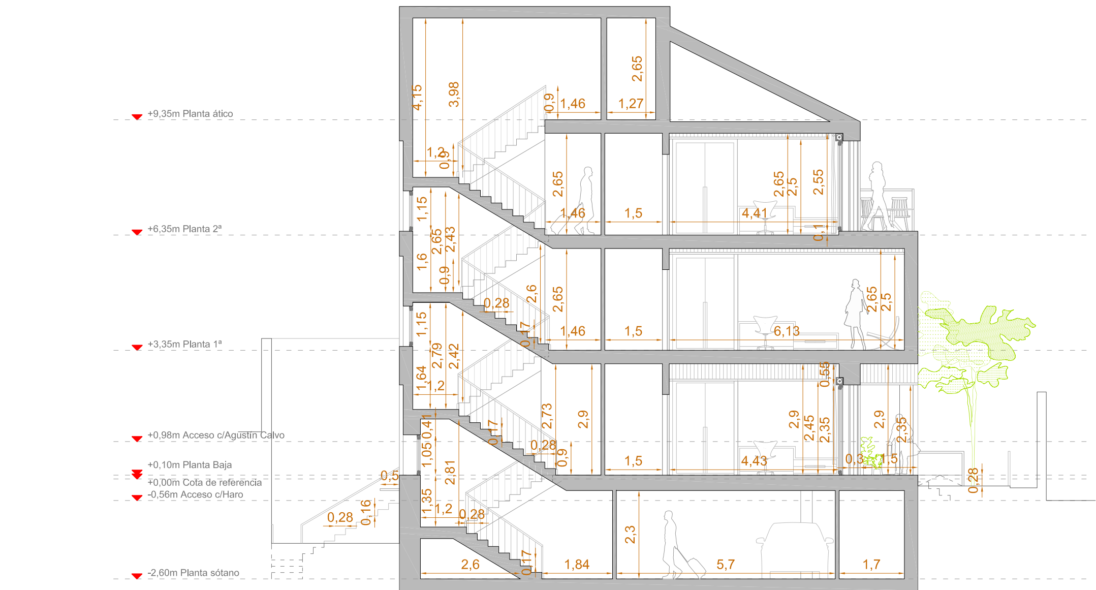
SECCIÓN 2
