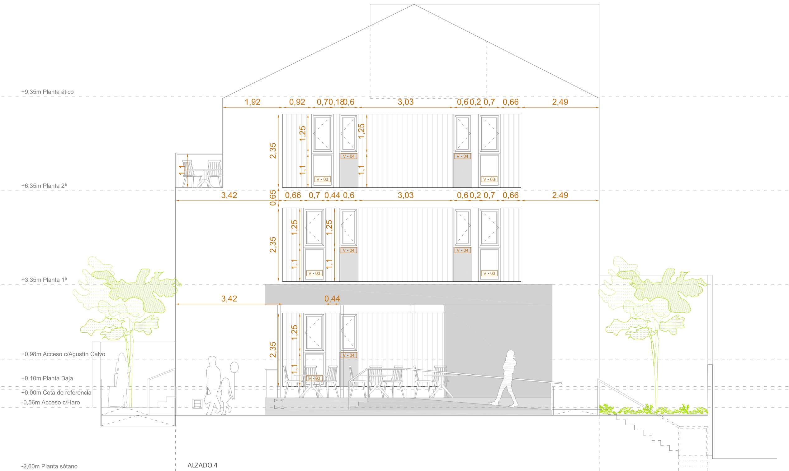
ALZADO 4
