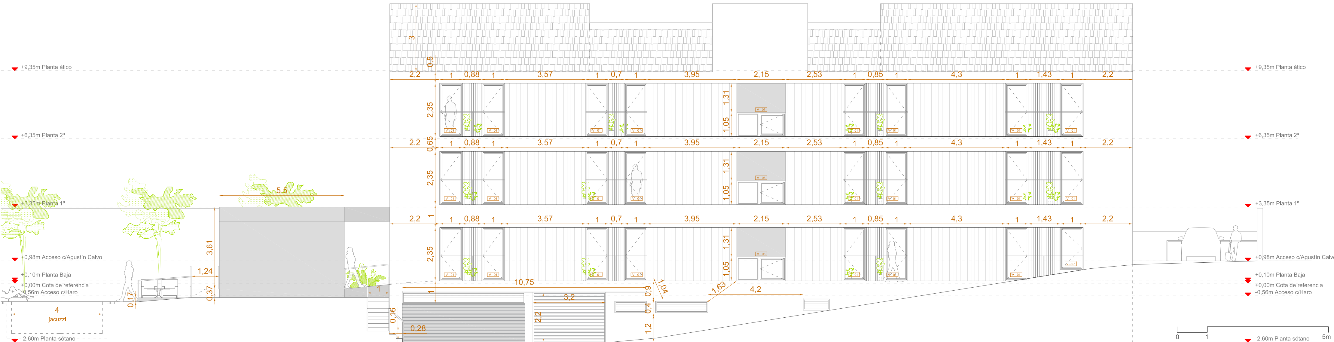
ALZADO 1
