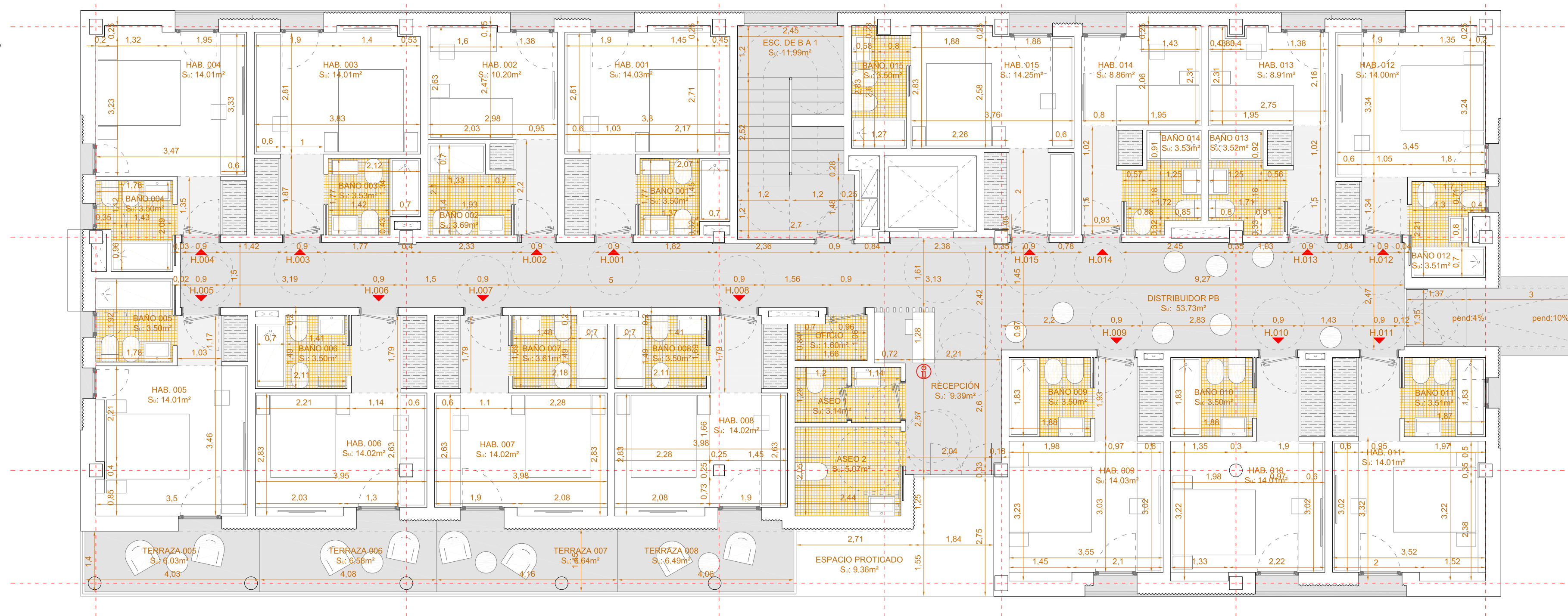
PLANTA BAJA
