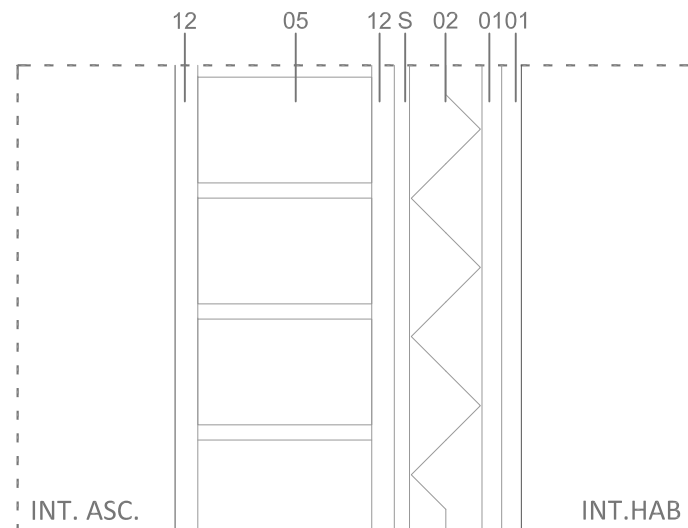
P05: PARTICIÓN ASCENSOR CON HABITACIONES
