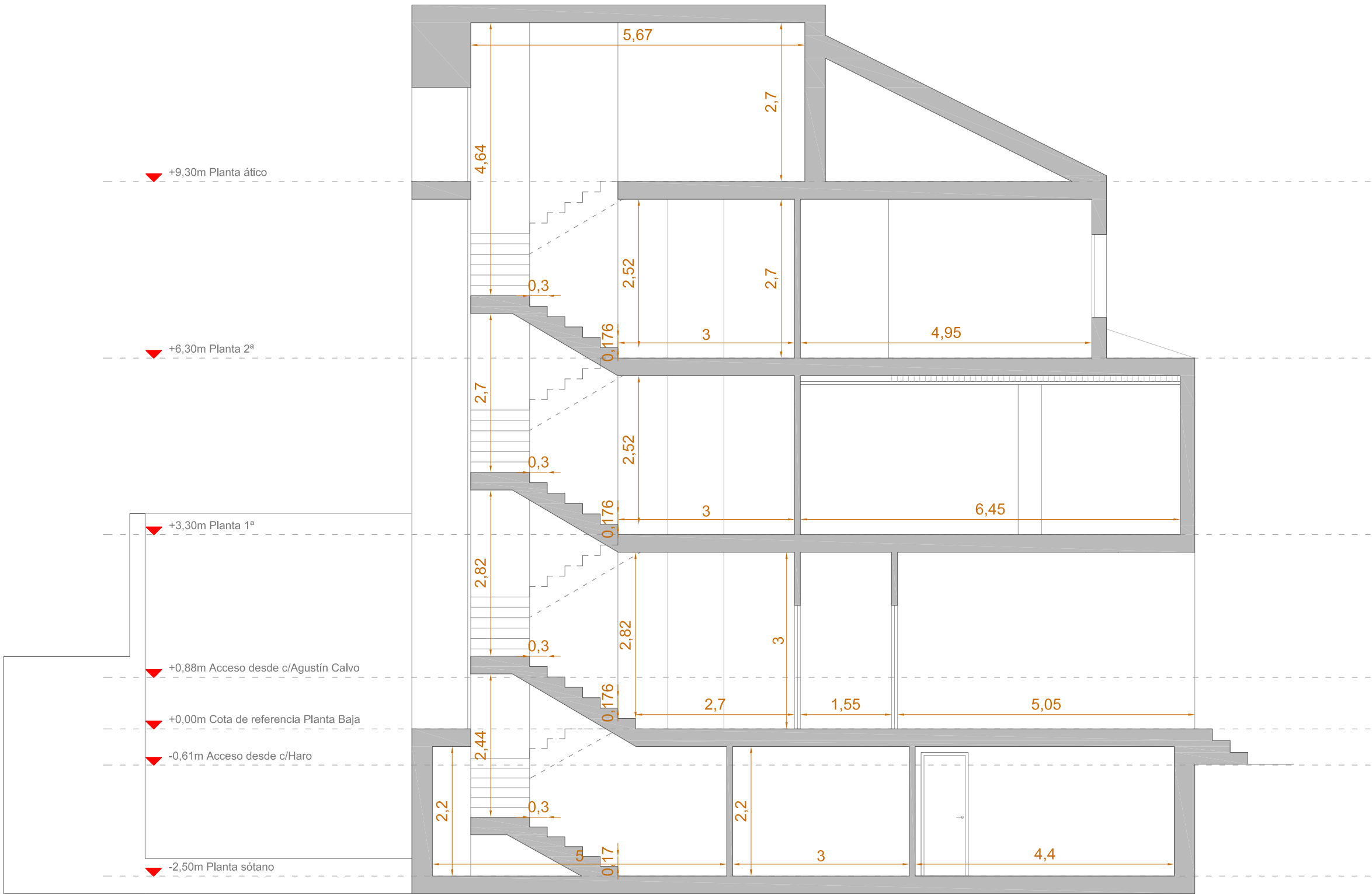
SECCIÓN 2
