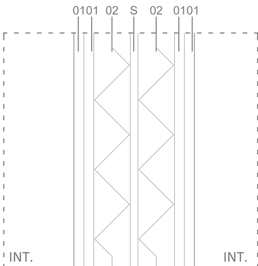
P01: PARTICIÓN ENTRE HAB. Y ENTRE HABITACIONES Y Z. COMUNES
