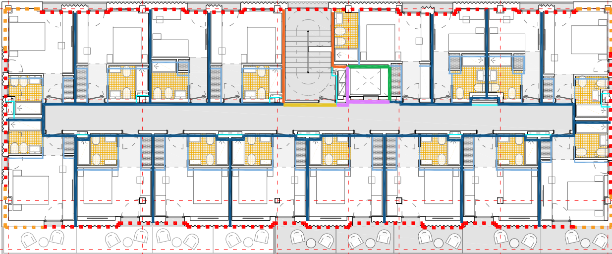
PLANTA 2ª
