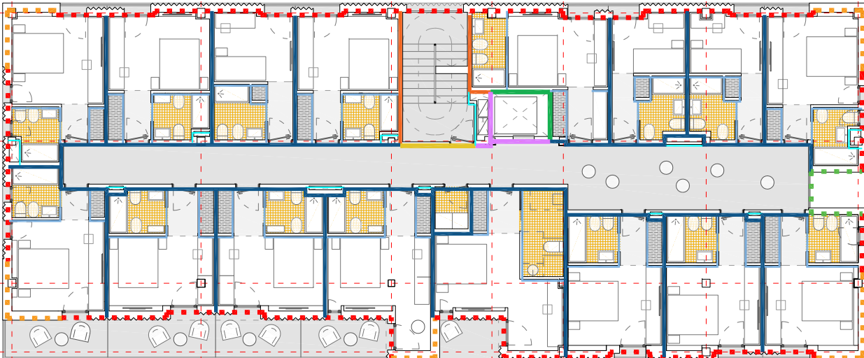
PLANTA 1ª
