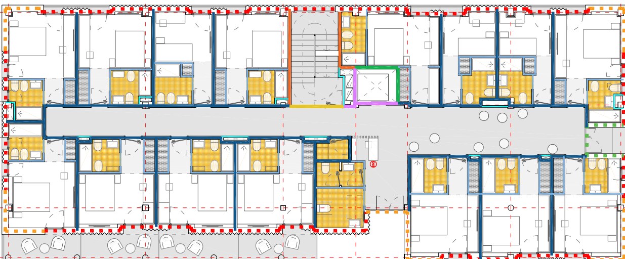
PLANTA BAJA
