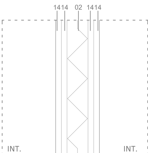
P06: PARTICIÓN INTERIOR ESCALERA CON DISTRIBUIDOR
