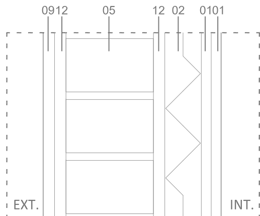
F04: FACHADA CASETÓN 2
