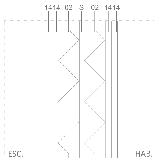
P08: PARTICIÓN ENTRE ESCALERA Y HABITACIONES
