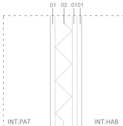
P03: PARTICIÓN ENTRE PATINILLOS Y HABITACIONES
