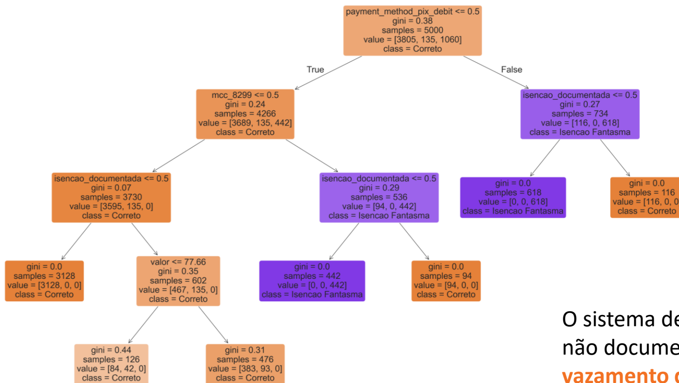
Árvore de Decisão: Regras Ocultas
