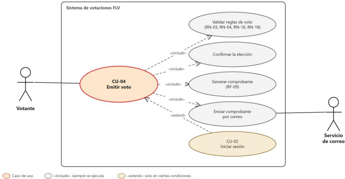
Figura 6 Diagrama del caso de uso CU-04 – Emitir voto
