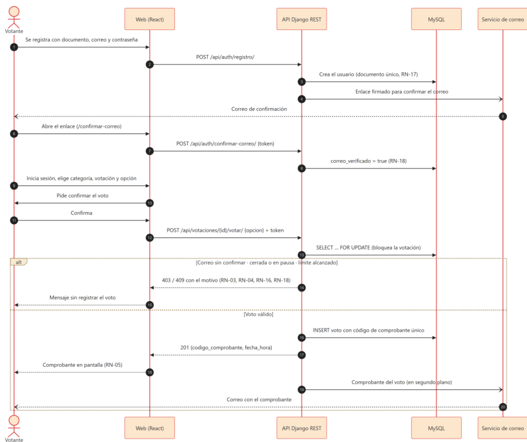
Figura 20 Diagrama de secuencia del flujo principal de votación
