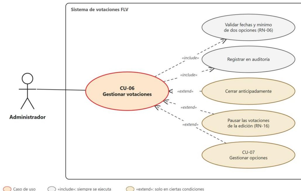
Figura 8 Diagrama del caso de uso CU-06 – Gestionar votaciones
