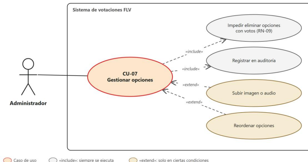
Figura 9 Diagrama del caso de uso CU-07 – Gestionar opciones
