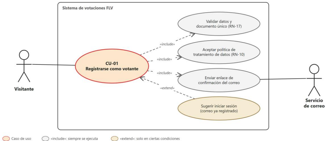
Figura 3 Diagrama del caso de uso CU-01 – Registrarse como votante
