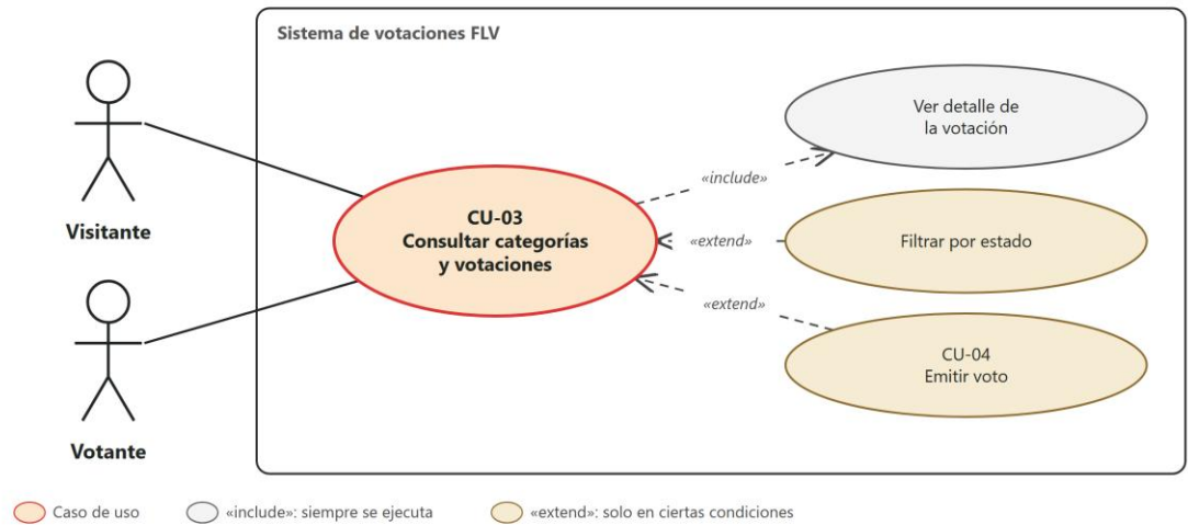
Figura 5 Diagrama del caso de uso CU-03 – Consultar categorías y votaciones
