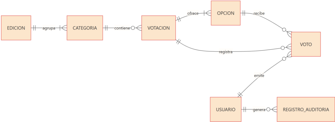
Figura 12 Modelo conceptual de datos: entidades, relaciones y cardinalidades
