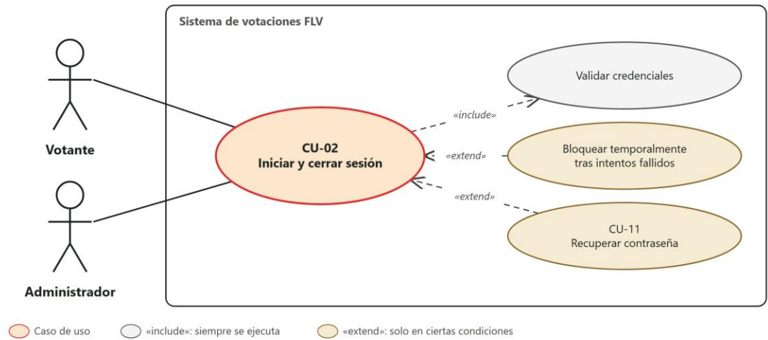
Figura 9 Diagrama del caso de uso CU-02 – Iniciar y cerrar sesión
