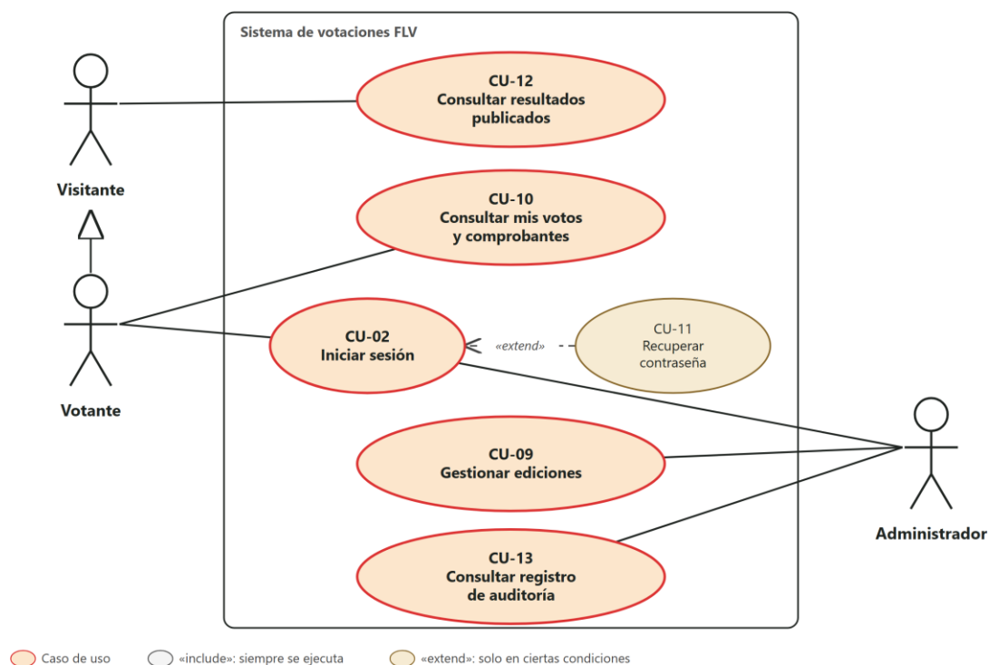
Figura 16 Diagrama de los casos de uso complementarios CU-09 a CU-13
