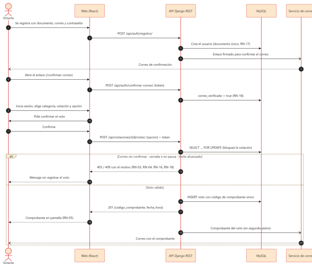
Figura 20 Diagrama de secuencia del flujo principal de votación
