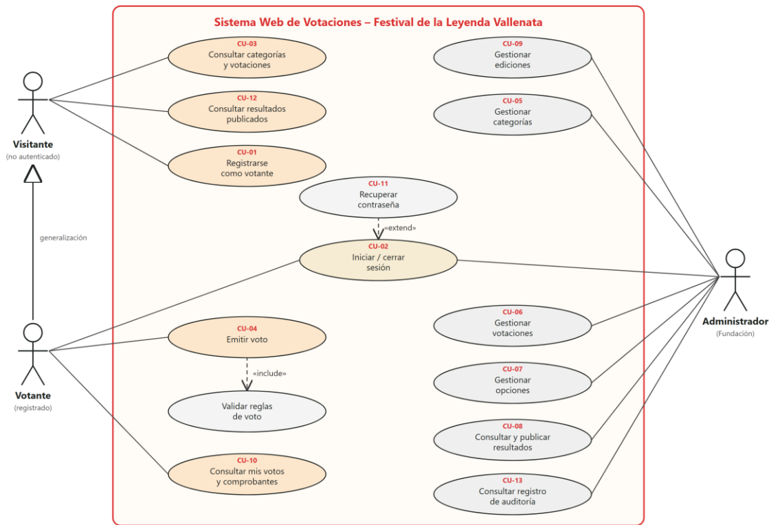
Figura 2 Diagrama general de casos de uso
