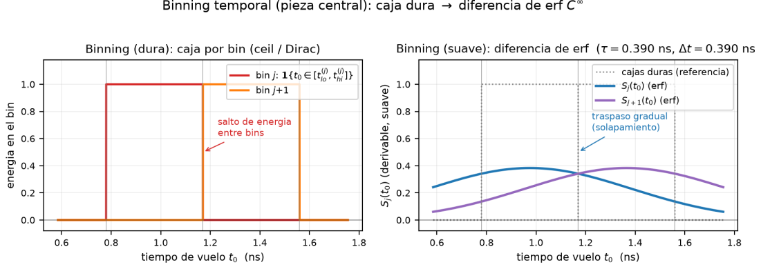
Figure 1: Binning temporal (paso (i), pieza central ). Izquierda: función no derivable (dura): la energía se deposita entera en una caja por bin ( \lceil \cdot \rceil / Dirac), de modo que salta de golpe del bin j al j+1 al cruzar el borde. Derecha: su reemplazo suave , la diferencia de erf (10) para los mismos dos bins: las curvas S_j, S_{j+1} se solapan y la energía se traspasa gradualmente (cajas duras punteadas de referencia). Parámetros reales \tau = \Delta t de ForwardConfig.
