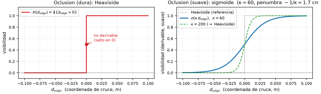
Figure 2: Ocultamiento (paso (ii)). Izquierda: función no derivable (dura): el Heaviside 1\{d_{\text{edge}} > 0\} , con salto en d_{\text{edge}} = 0 . Derecha: su reemplazo suave , la sigmoide \sigma(\kappa d_{\text{edge}}) (12) con \kappa = 60 (penumbra \sim 1/\kappa ); una segunda curva con \kappa = 200 sugiere el límite \kappa \rightarrow \infty (Heaviside punteado de referencia). Parámetro real de ForwardConfig .
