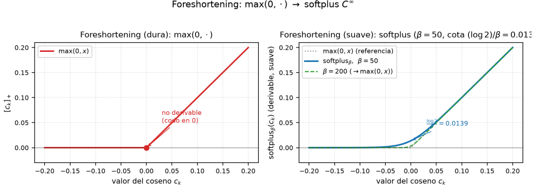
Figure 3: Foreshortening (paso (iii)). Izquierda: función no derivable (dura): el clamp \max(0, c_k) , con codo no derivable en c_k = 0 . Derecha: su reemplazo suave , la \text{softplus}_\beta(c_k) (13) con \beta = 50 ; se anota la cota uniforme (\log 2)/\beta (Prop. 14) y una segunda curva con \beta = 200 sugiere el límite \beta \rightarrow \infty ( \max(0, \cdot) ) punteado de referencia). Parámetro real de ForwardConfig .
