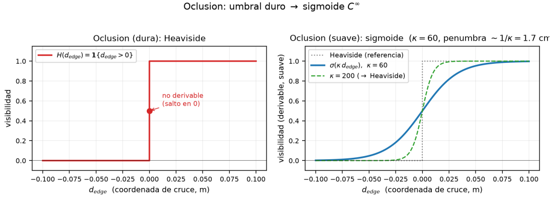
Figure 2: Ocultamiento (paso ii). Izquierda: función no derivable (dura): el Heaviside \mathbf{1}\{d_{\text{edge}} > 0\} , con salto en d_{\text{edge}} = 0 . Derecha: su reemplazo suave , la sigmoide \sigma(\kappa d_{\text{edge}}) (12) con \kappa = 60 (penumbra \sim 1/\kappa ); una segunda curva con \kappa = 200 sugiere el límite \kappa \rightarrow \infty (Heaviside punteado de referencia). Parámetro real de ForwardConfig .
