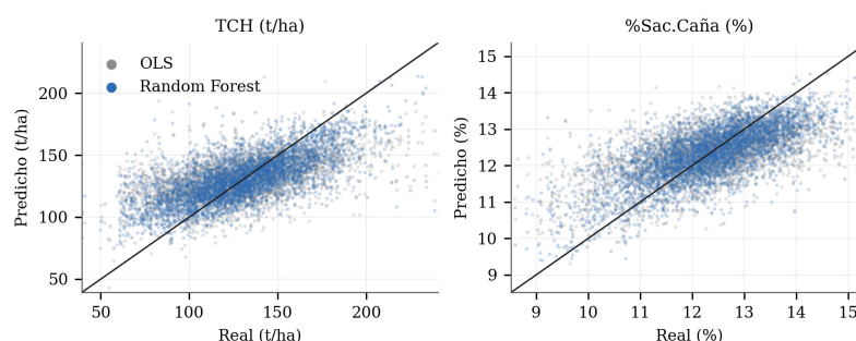
Fig. 1. Valores reales frente a predichos en el conjunto de prueba (OLS en gris, Random Forest en azul). Ambos modelos comprimen los extremos hacia la media.
