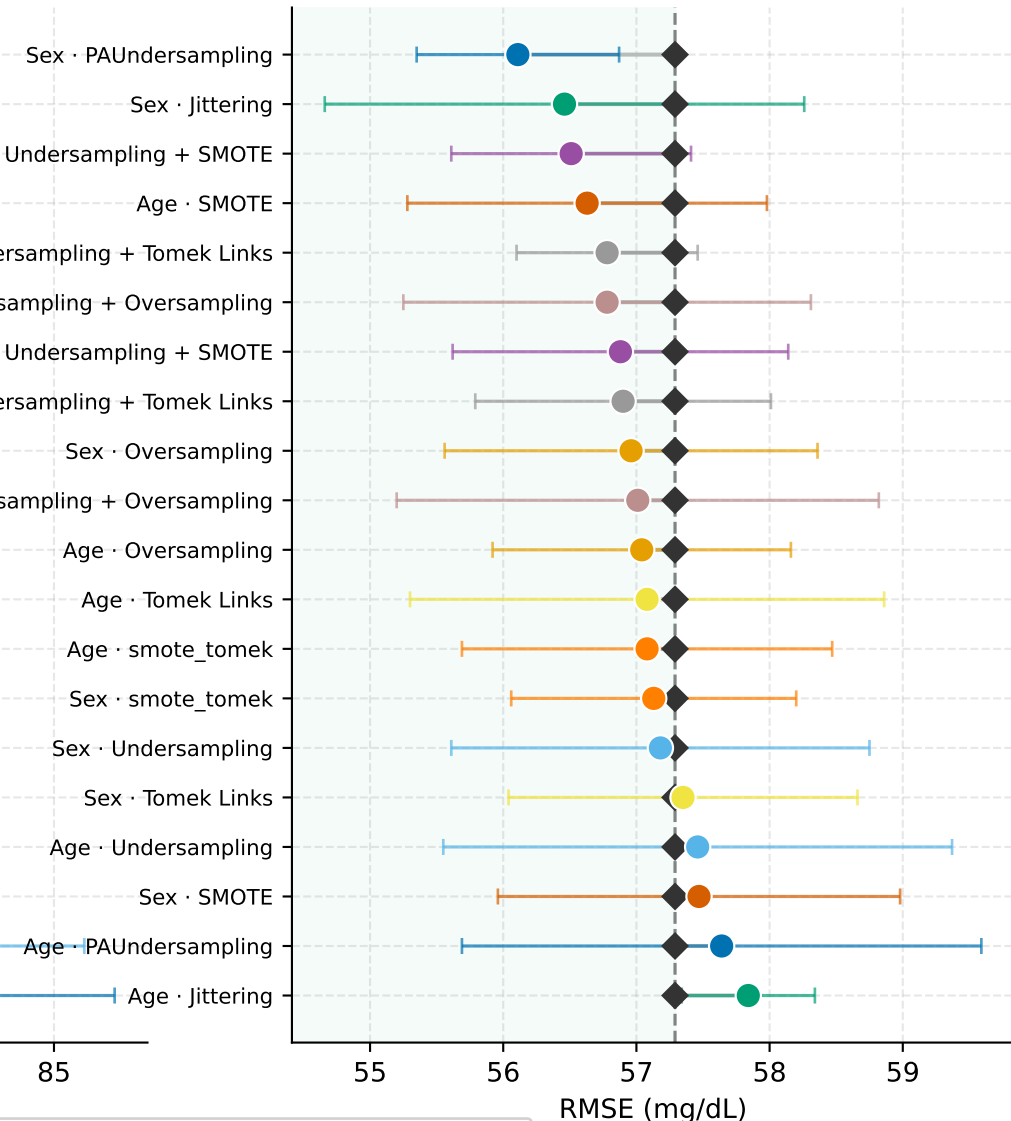
ReplaceBG
