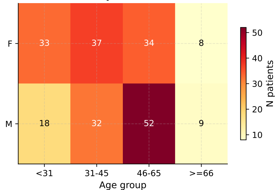
ReplaceBG
