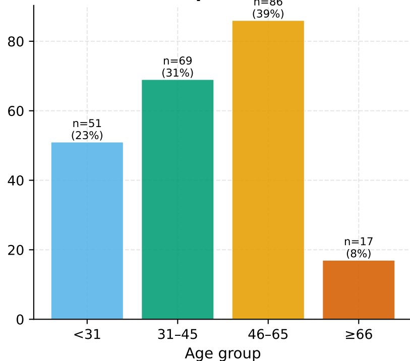
ReplaceBG
