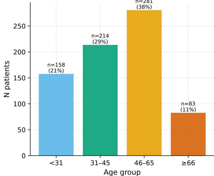
T1DiabetesGranada
