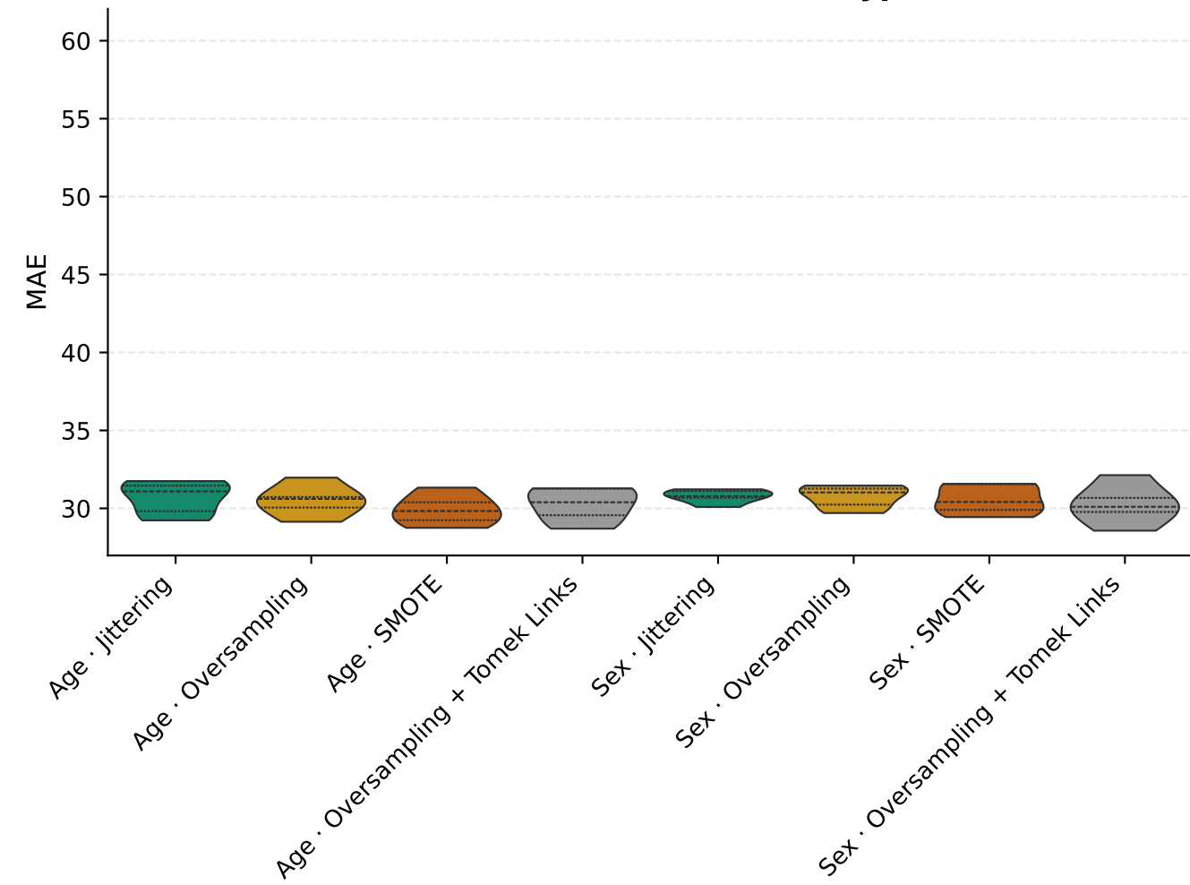
T1DiabetesGranada — MAE · Hypo L1
