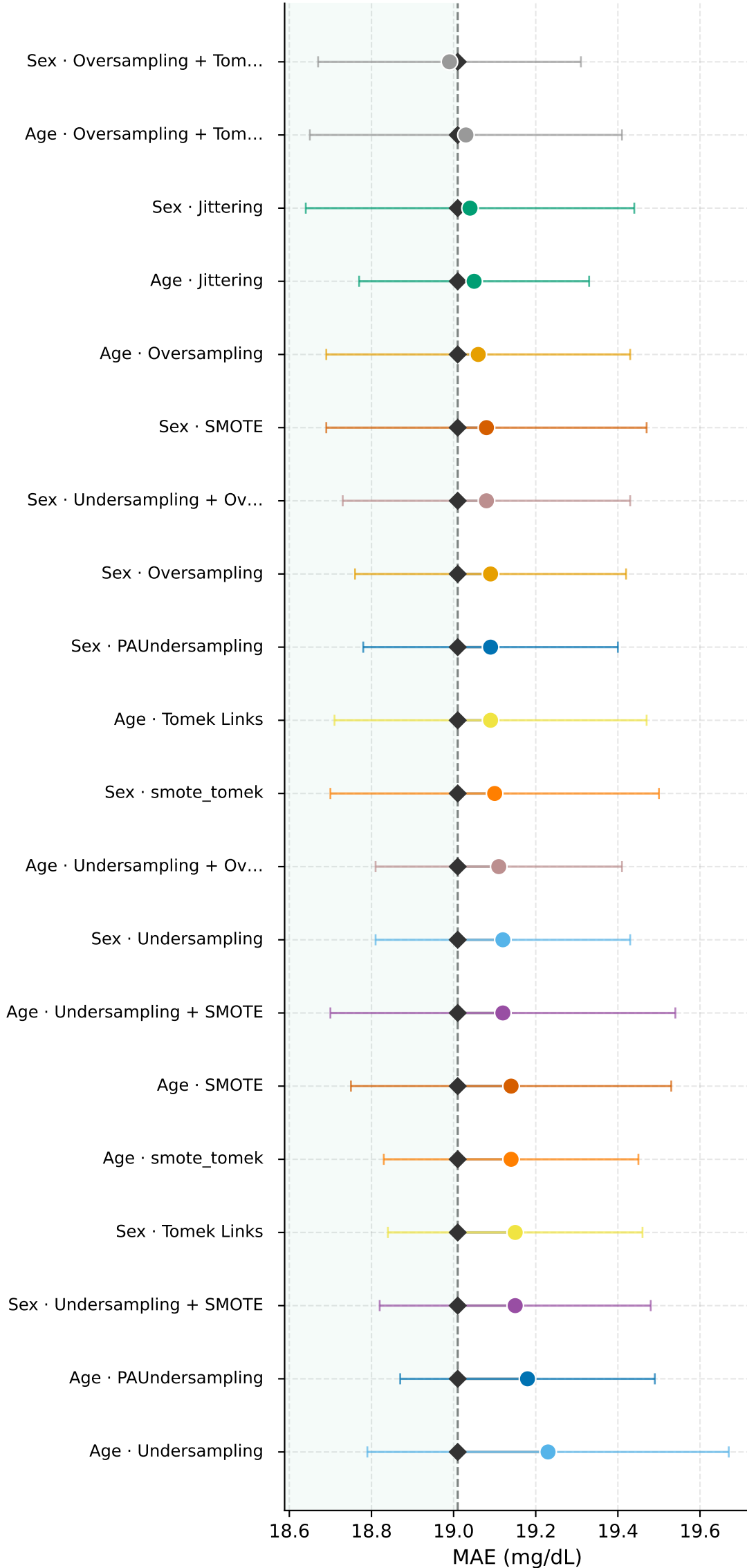
ReplaceBG
