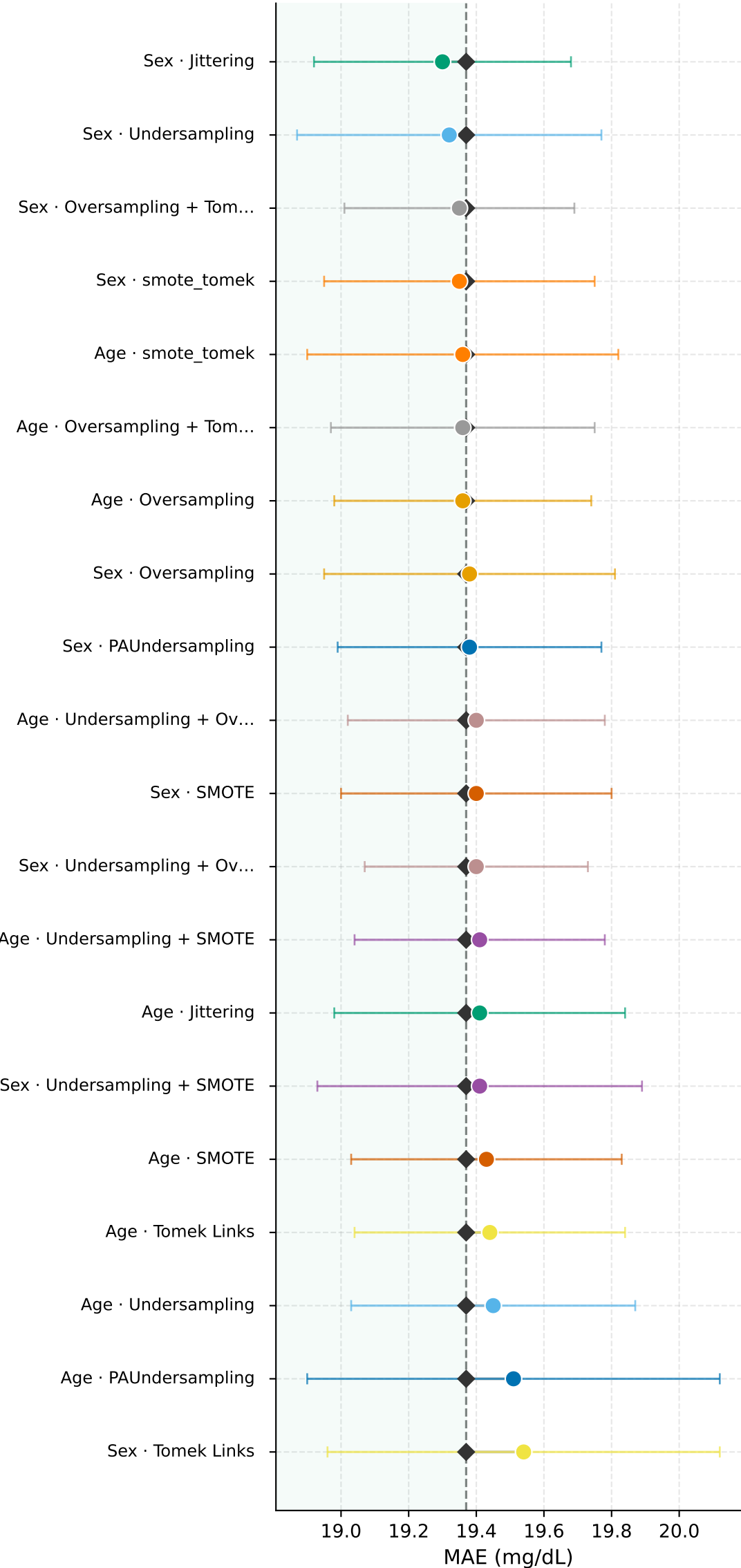
T1DiabetesGranada
