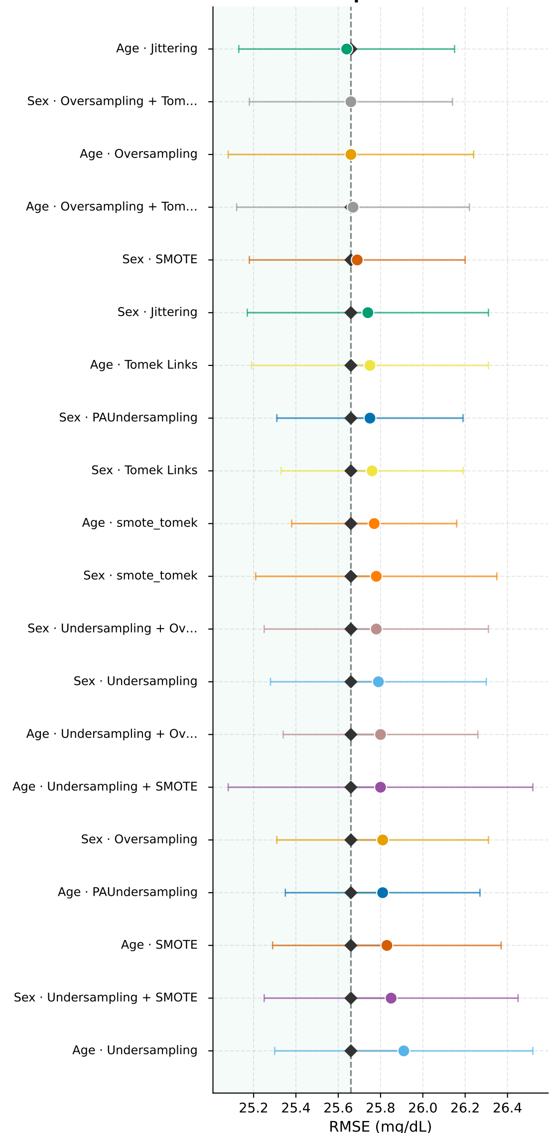
ReplaceBG
