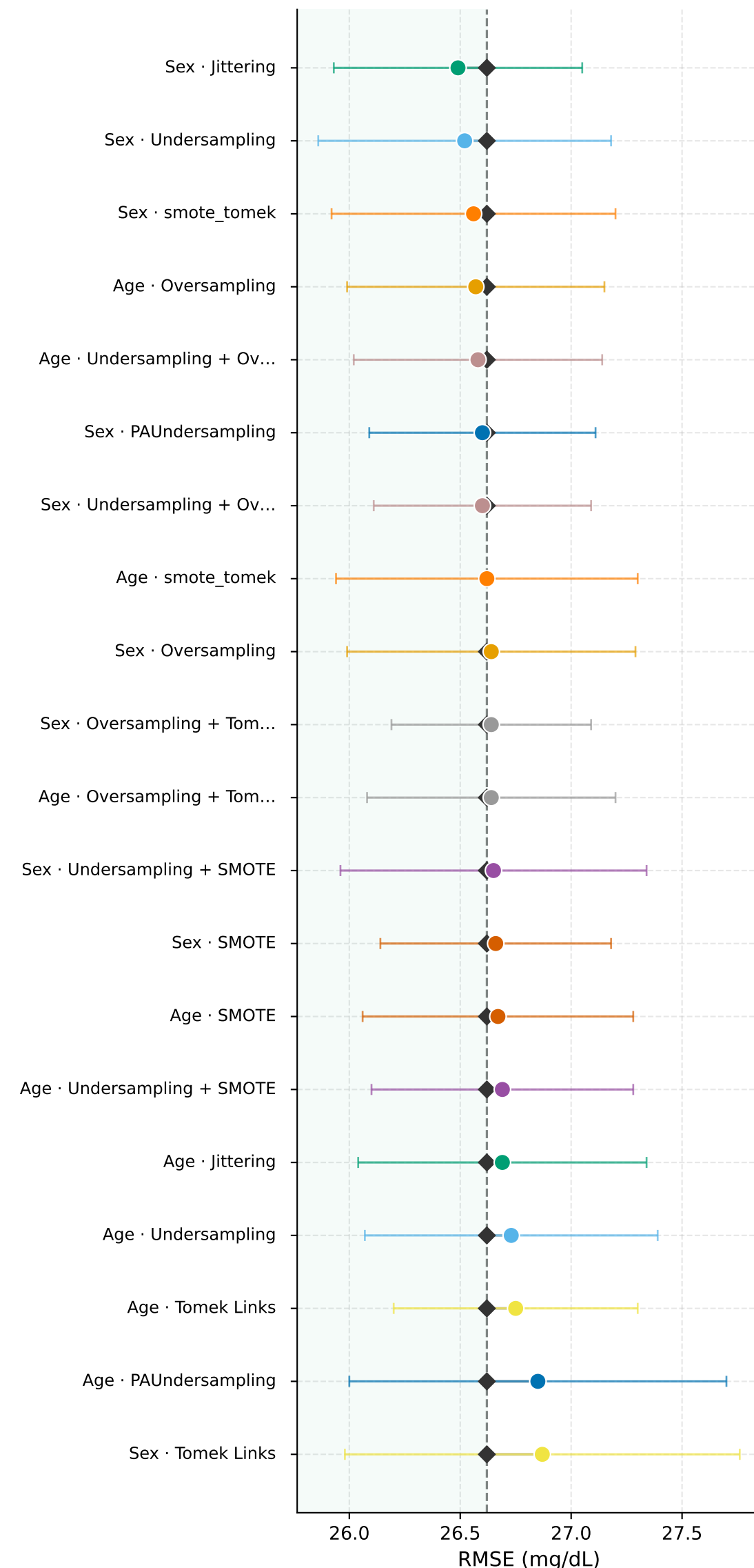
T1DiabetesGranada
