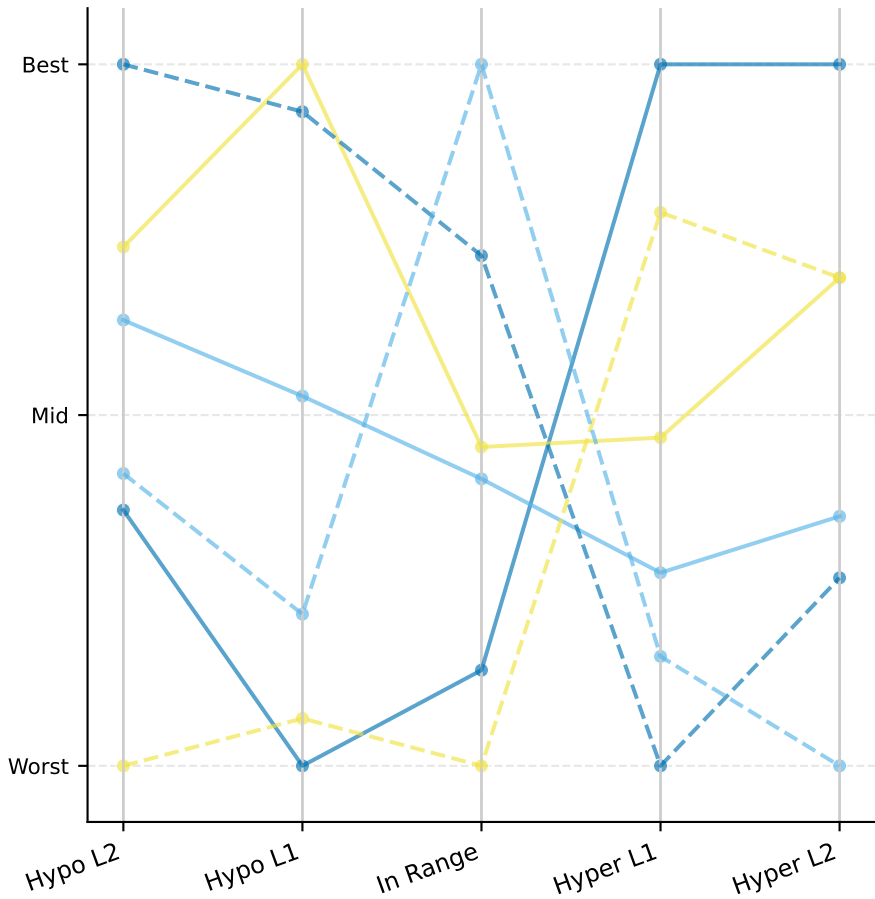
T1DiabetesGranada
