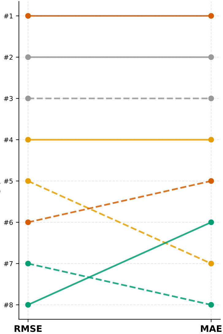
T1DiabetesGranada
