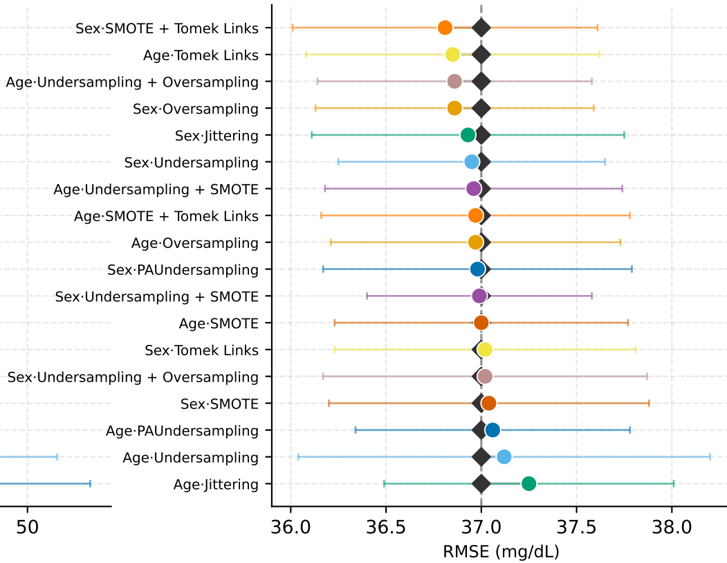
ReplaceBG Dumbbell: RMSE·All ranges
