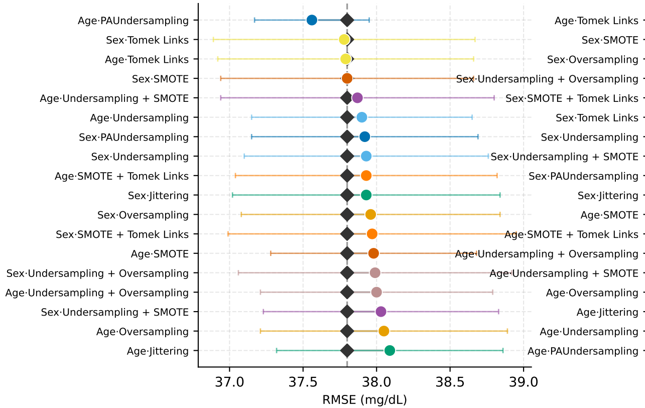
T1DGranada Dumbbell: RMSE·All ranges
