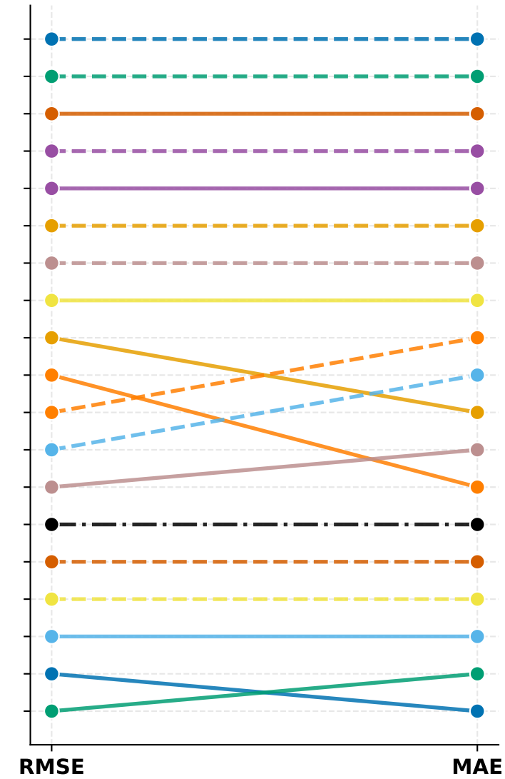
ReplaceBG
