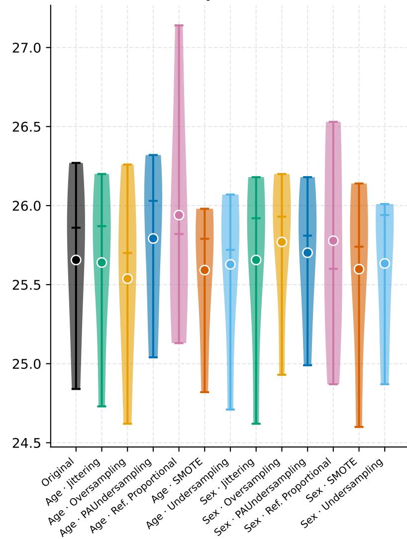
ReplaceBG
