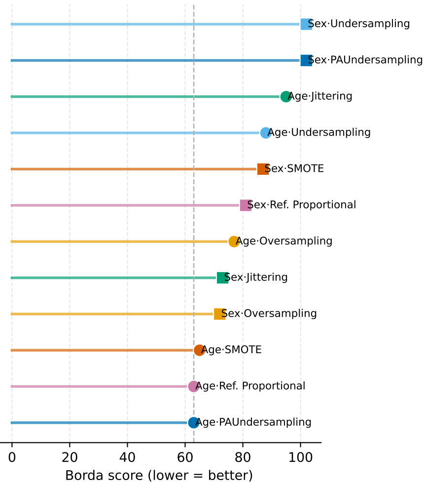
ReplaceBG
