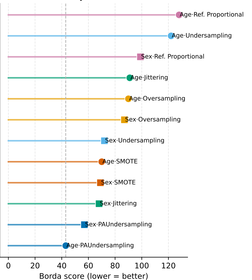
ReplaceBG
