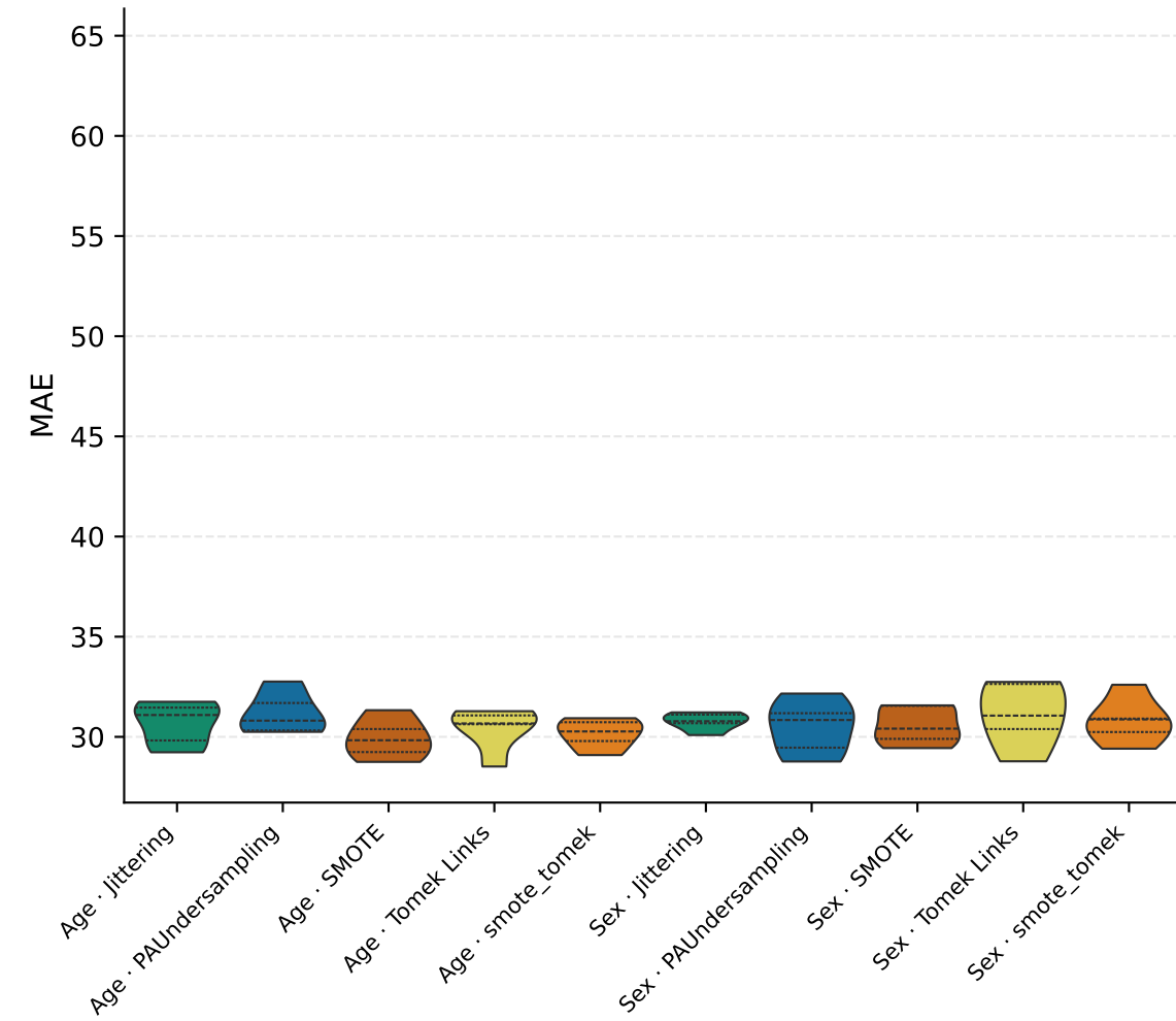
T1DiabetesGranada — MAE · Hypo L1
