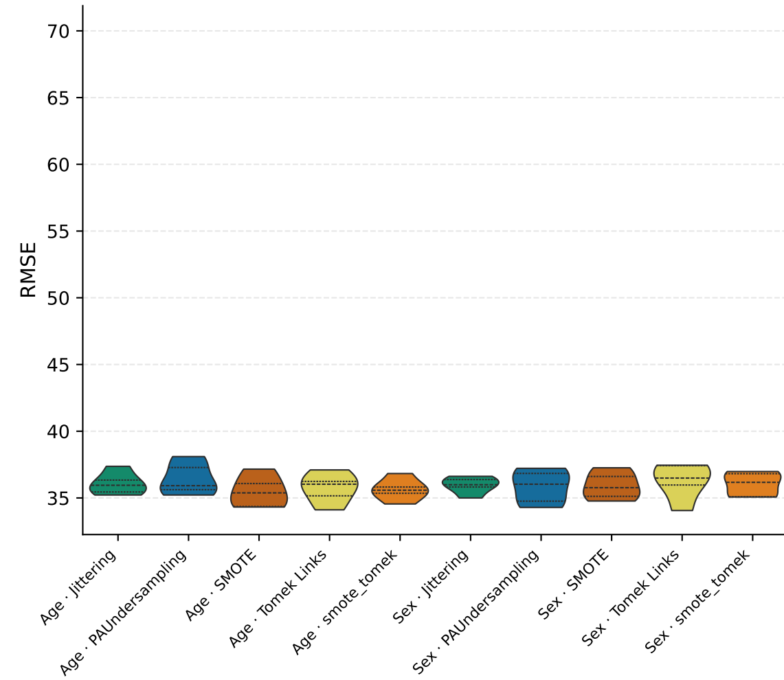
T1DiabetesGranada — RMSE · Hypo L1
