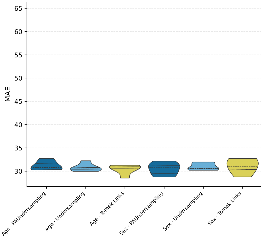
T1DiabetesGranada — MAE · Hypo L1
