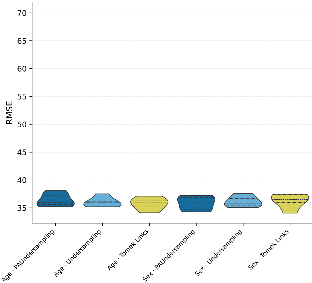
T1DiabetesGranada — RMSE · Hypo L1
