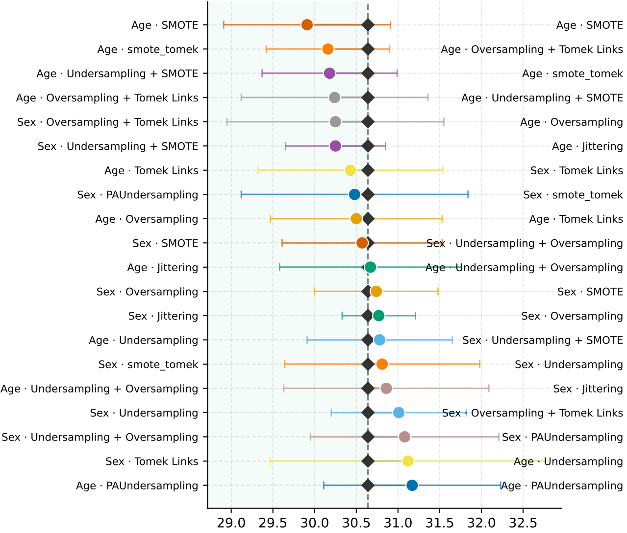
T1DiabetesGranada
