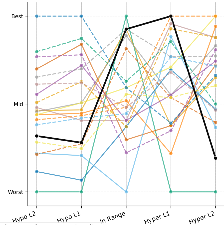
ReplaceBG
