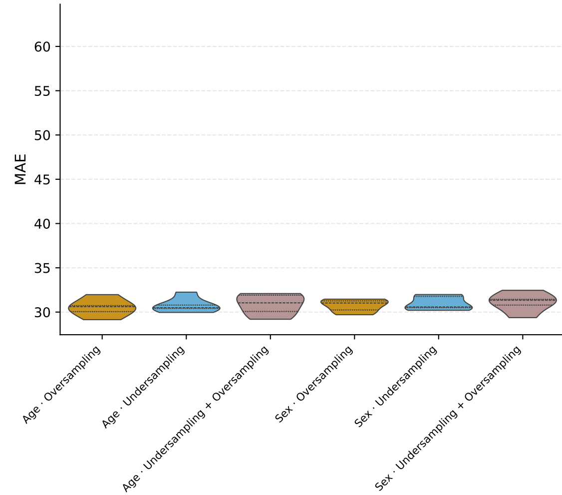
T1DGranada — MAE · Hypo L1
