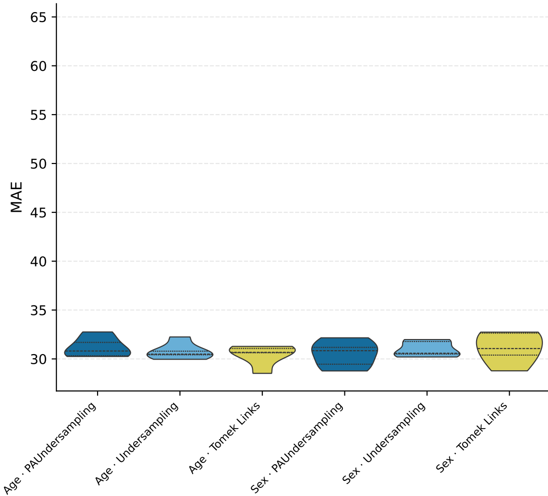
T1DGranada — MAE · Hypo L1
