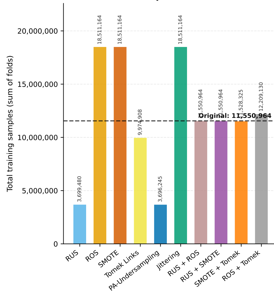
ReplaceBG
