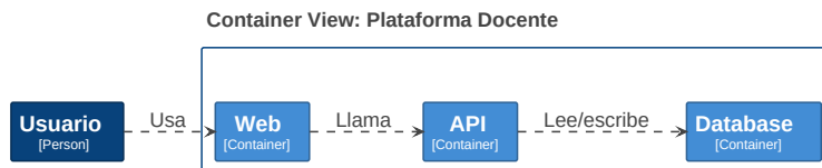
Figura9.6: Diagrama: Structurizr: vista C4 simplificada.
