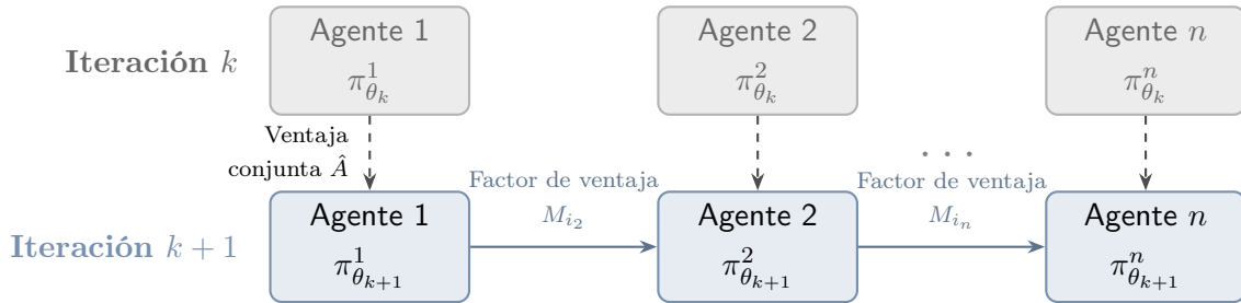
Figura 2.20: Esquema de actualización secuencial de HAPPO. A diferencia de PPO independiente, la actualización de cada agente está condicionada por el factor de ventaja ponderada M_{i_m} , que incorpora los cambios efectuados por los agentes que lo precedieron en la secuencia.
