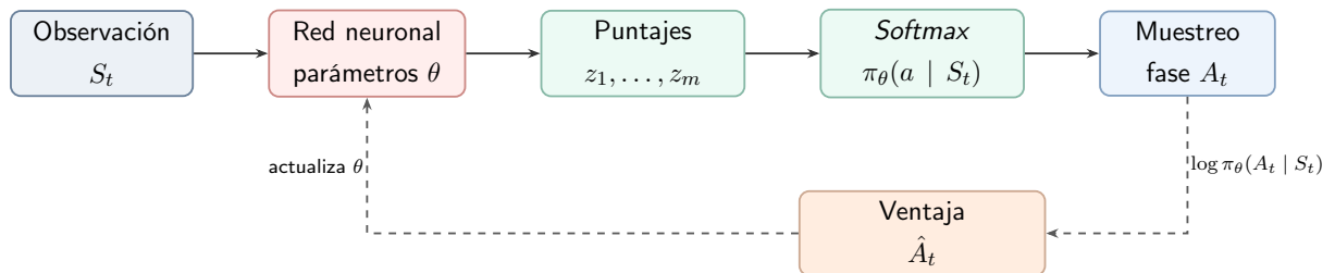
Figura 2.15: Red de política para un espacio discreto de fases. La observación determina una distribución de acciones; durante el aprendizaje, la ventaja pondera el gradiente de la log-probabilidad de la acción seleccionada [SB18, KT03].
