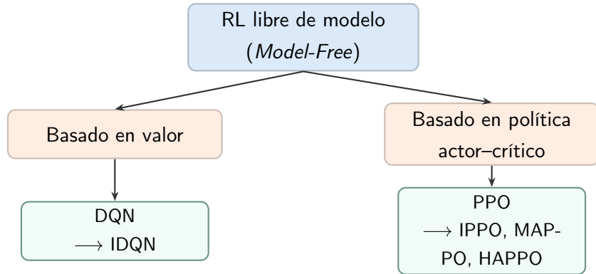
Figura 2.11: Relación entre las familias de algoritmos utilizadas en esta investigación. Los cuatro métodos evaluados son libres de modelo y se derivan de las líneas DQN y PPO.
