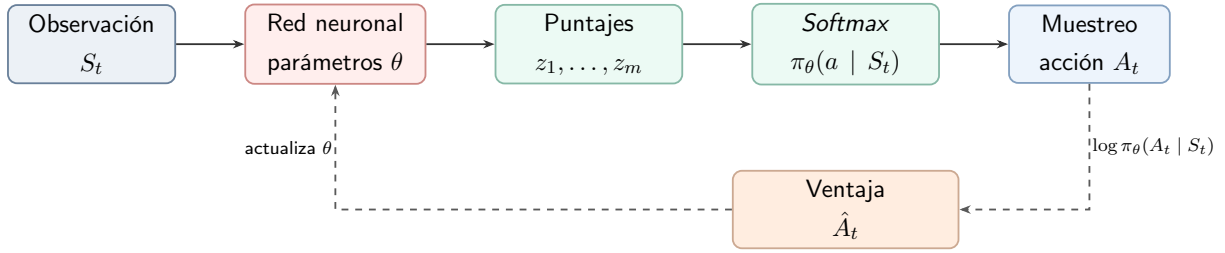
Figura 2.16: Red de política para un espacio discreto de acciones. La observación determina una distribución sobre las acciones disponibles; durante el aprendizaje, la ventaja pondera el gradiente de la log-probabilidad de la acción seleccionada [SB18, KT03].
