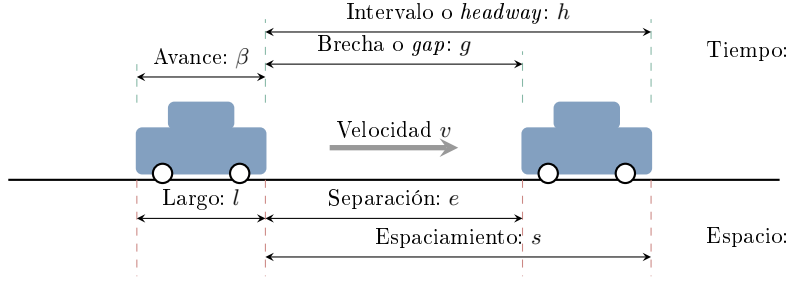
Figura 2.2: Relaciones temporales y espaciales entre vehículos consecutivos de una corriente de tránsito: intervalo ( h ) y espaciamiento ( s ).
