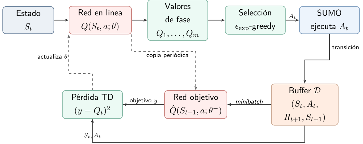
Figura 2.15: Flujo conceptual de DQN con repetición de experiencias y red objetivo. La red en línea selecciona acciones y recibe las actualizaciones; la red objetivo proporciona el término de bootstrapping del blanco TD. Elaboración propia a partir del algoritmo descrito por Mnih et al. [MKS + 15].
