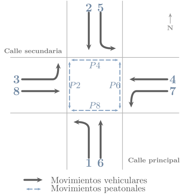
Figura 2.1: Convención esquemática de movimientos vehiculares, fases y cruces peatonales concurrentes en una intersección de cuatro accesos, adaptada conceptualmente del manual de temporización semafórica de Administración Federal de Carreteras ( Federal Highway Administration ) (FHWA) [Fed08].
