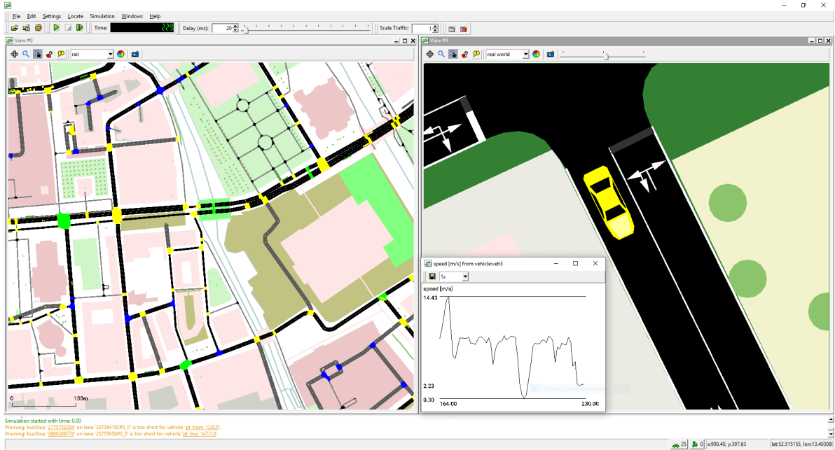
Figura 2.7: Interfaz gráfica de SUMO durante la ejecución de una simulación microscópica, con visualización de la red y de variables del vehículo.
