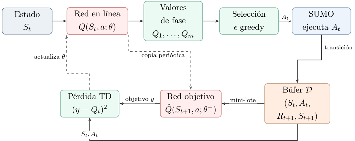
Figura 2.14: Flujo conceptual de DQN con repetición de experiencias y red objetivo. La red en línea selecciona acciones y recibe las actualizaciones; la red objetivo proporciona el término de bootstrapping del blanco TD. Elaboración propia a partir del algoritmo descrito por Mnih et al. [MKS + 15].
