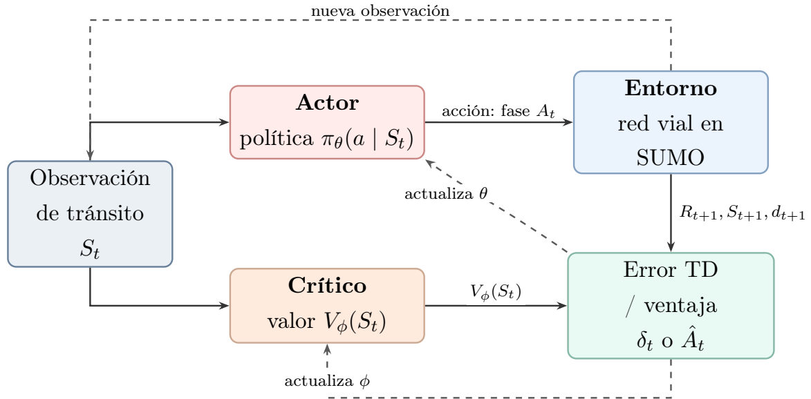
Figura 2.10: Arquitectura actor-crítico aplicada al control semafórico. El actor selecciona una acción y el crítico evalúa la transición para construir la señal que actualiza ambos componentes. Elaboración propia a partir de [KT03, SB18].
