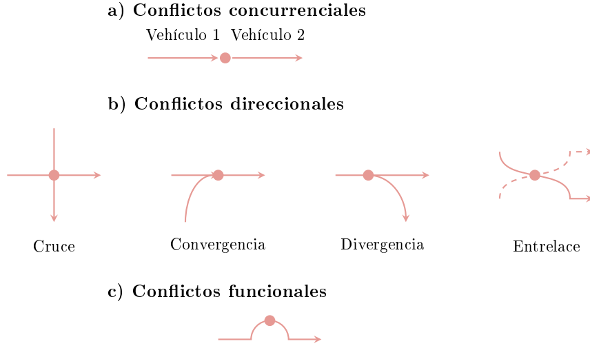
Figura 2.1: Representación esquemática de movimientos vehiculares y puntos de conflicto en una intersección semaforizada.
