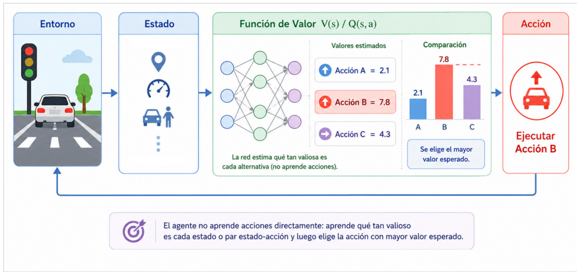
Figura 2.10: Esquema de un método basado en valor. A partir del estado observado s , una función de valor estima el retorno esperado, ya sea sobre estados V(s) o sobre pares estado–acción Q(s, a) . En el caso mostrado, las estimaciones para las acciones disponibles se comparan y se selecciona la alternativa con mayor valor esperado para ejecutarla en el entorno. La exploración puede incorporarse mediante estrategias como la selección \epsilon -codiciosa [SB18].
