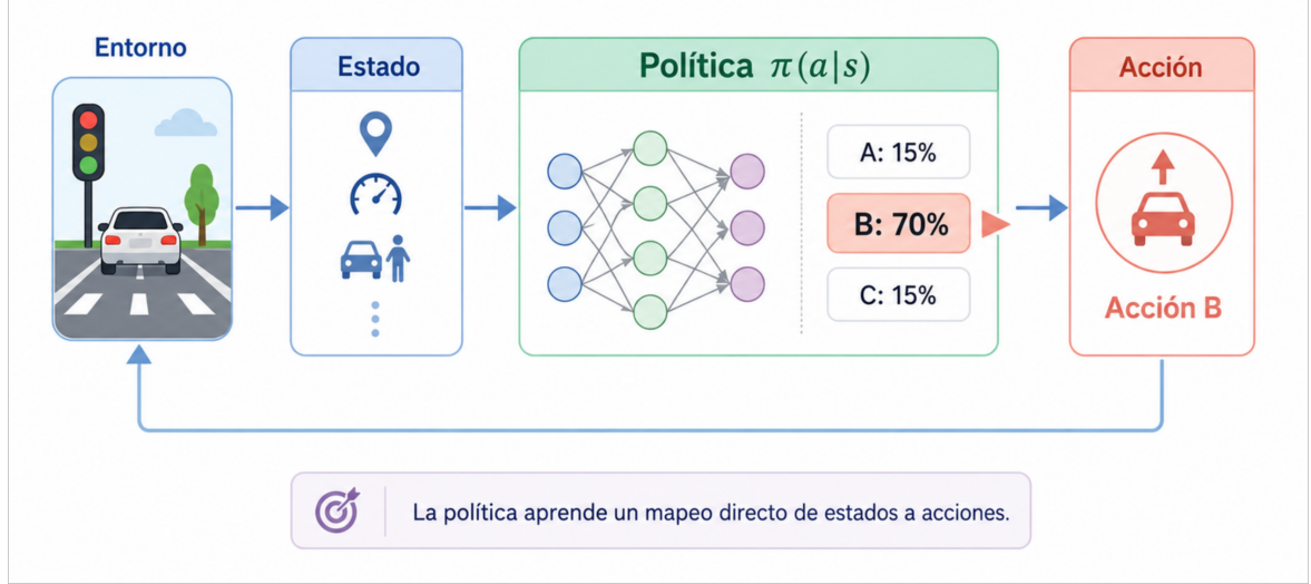
Figura 2.11: Esquema de un método basado en política. A partir del estado observado s , la política parametrizada \pi_\theta(a | s) , representada mediante una red neuronal, produce una distribución de probabilidad sobre las acciones disponibles. En el ejemplo, la acción B recibe la mayor probabilidad; la regla de ejecución puede seleccionarla directamente o muestrear una acción de la distribución [Hugnd].
